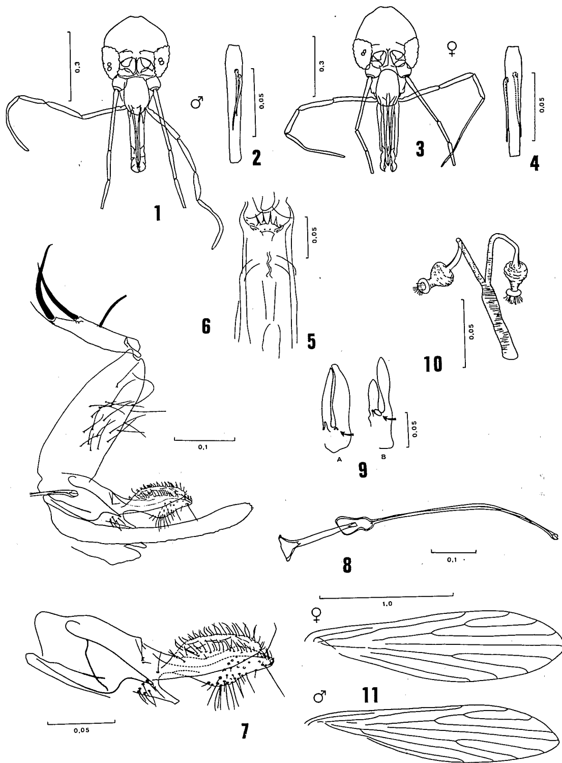
Fig. 1-11. — Lutzomyia torresi n. sp., holotype mâle et allotype femelle. — 1, tête du mâle ; 2, flagellomère antennaire A IV, 3, tête de la femelle ; 4, flagellomère antennaire IV de la femelle ; 5, cibarium ; 6, genitalia ; 7, paramère ; 8, pompe et filaments génitaux ; 9 : paramère en vue ventrale (A : L. torresi ; B : L. boliviana ; la flèche indique la zone d'insertion des soies) ; 10, spermatheques ; 11, aile.
