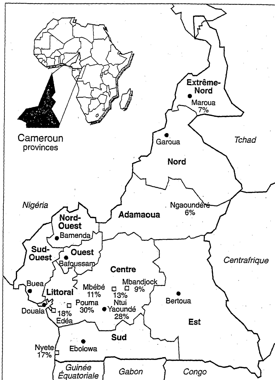
Figure 1. Variations géographiques des taux de chloroquinorésistance de P. falciparum évalués par tests in vivo (1989-1991).
