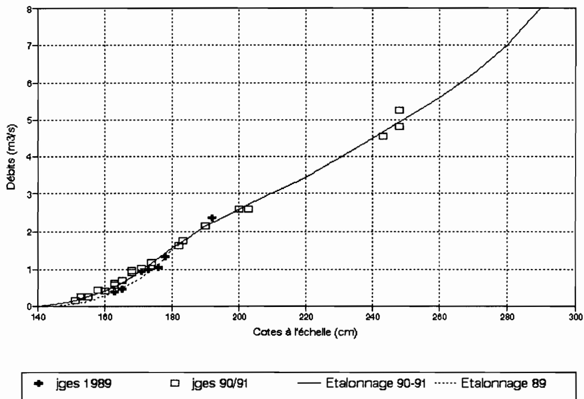
ETALONNAGE DE LA CRIQUE TOUSSAINT Courbe de basses et moyennes eaux
