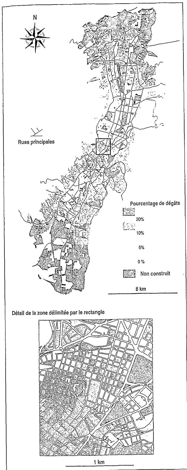
4c. Distribution des dommages subis par les bâtiments de Quito pour le séisme local
