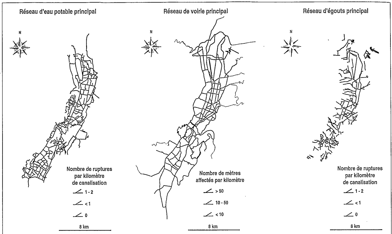
5. Distribution des dommages subis par Quito pour le séisme local par le réseau de distribution d'eau potable (gauche) — par le réseau de voirie (centre) — par le réseau des égouts (droite)
