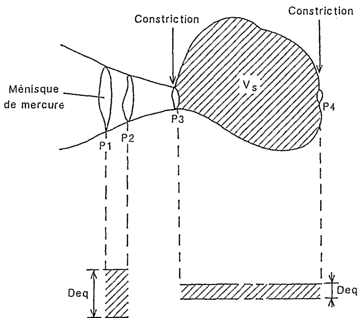
Progression du mercure dans un pore en fonction de la pression appliquée
