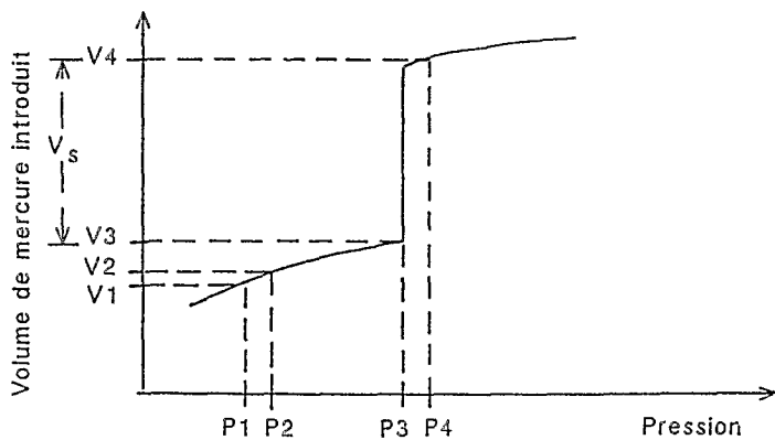
Courbe du volume de mercure introduit en fonction de la pression appliquée
