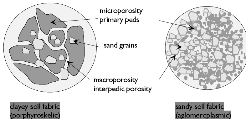
figure 6 : modèle morphologique de la structure du sol à ses deux premiers niveaux d'organisation
