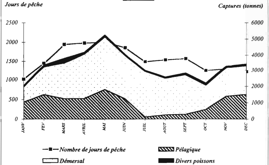
Evolution mensuelle du nombre de jours de pêche et des captures
