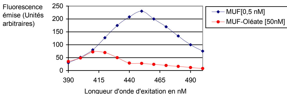
Figure 8- Spectre d'émission MUF-Oléate / MUF après excitation à 365 nm. On observe pas de recouvrement des spectres à la longueur d'émission du MUF \lambda=450\text{nm} ).
