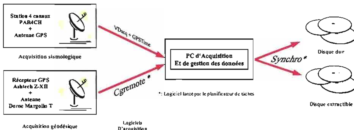
Fig . 6 : Schéma fonctionnel
