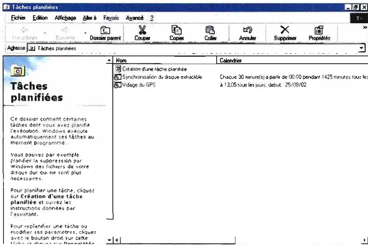
Fig . 5 : Les fichiers de commande gérés par le planificateur de tâches
