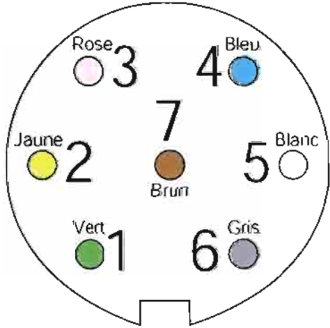
Prise mâle Amphenol Ref: T3104 101 vue ct soudures (vers PC).
