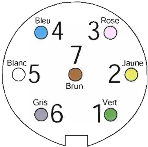
Prise femelle Amphenol Ref: T3105 101 vue ct soudures (vers Viseis).
