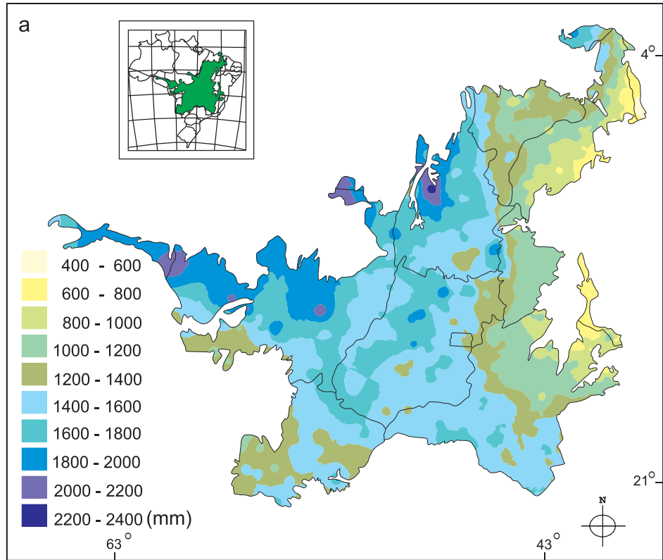
Figure 2 - Précipitations (a) et températures (b) moyennes annuelles du Cerrado.
