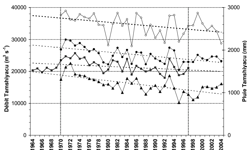
Fig. 7 Rio Amazonas à Tamshiyacu: Variabilité interannuelle des pluies (■) et des débits moyens (●), minimum (▲) et maximum (○) pour la période 1964-2005. Les courbes de tendance correspondent à la période commune 1970-2005.
