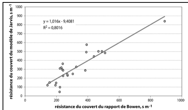
Figure 3 : Relation entre la résistance du couvert de la savane à Loudetia arundinacea issue du modèle de Jarvis-Stewart (Founa-Toutou, 2000) et du rapport de Bowen ; valeurs journalières lors de la période du 18 septembre au 11 octobre 1998. Relationship between the canopy resistance of savannah with Loudetia arundinacea obtained from Jarvis-Stewart model (Founa-Toutou, 2000) and from Bowen-ratio method; daily values during the period from September 18 to October 11, 1998.
