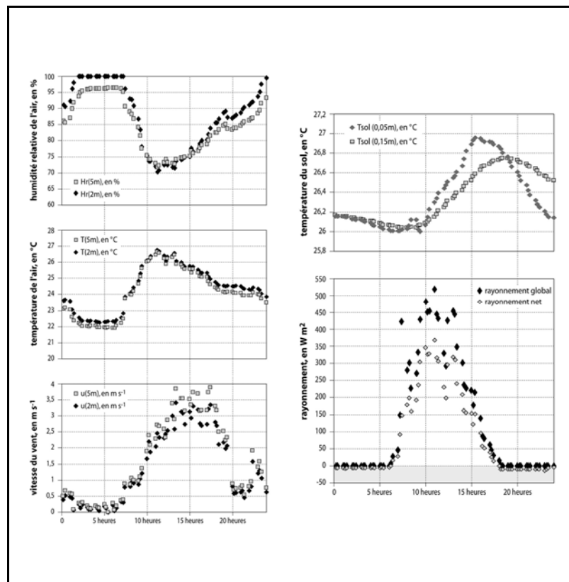
Figure 1 : Evolution au cours de la journée du 29 septembre 1998 (à gauche) de la température moyenne de l'air ( T_{air} ), de l'humidité relative de l'air ( Hr ), de la vitesse du vent ( u ) à 2,0 et 5,0 m au-dessus de la surface du sol de la savane ; (à droite) de la température du sol à 0,05 et 0,15 m de profondeur, du rayonnement global ( R_g ) et rayonnement net ( R_n ) à 6,0 m au dessus de la surface du sol de la savane. Evolution during the day of September 29, 1998 (a) of the mean air temperature ( T_{air} ), relative humidity ( Hr ), wind speed ( u ) 2.0 and 5.0 m above the soil surface of the savannah; (b) mean soil temperature at a depth of 0.05 m and 0.15 m; of global ( R_g ) and net radiation ( R_n ) at 6.0 m above the soil surface of the savannah.
