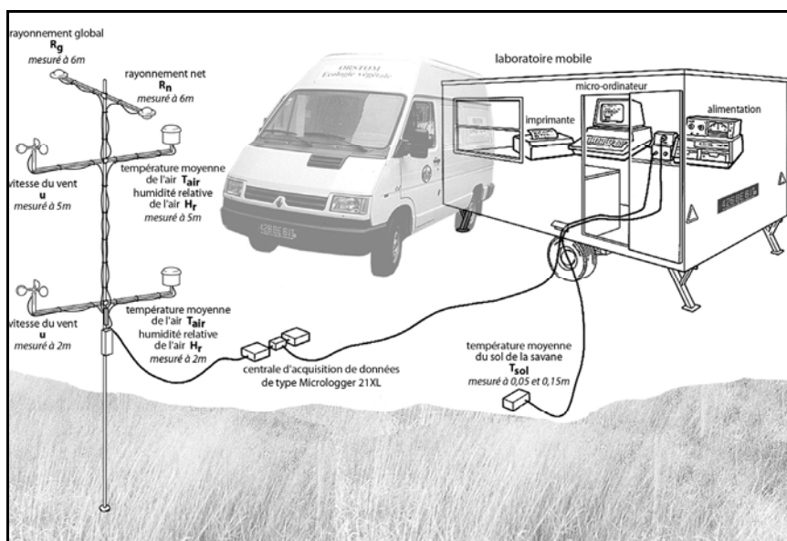
Figure 2 : Schéma du dispositif expérimental de mesure de l'évapotranspiration réelle d'un couvert végétal. Diagram of the experimental mobile laboratory of measurement of actual canopy evapotranspiration.
