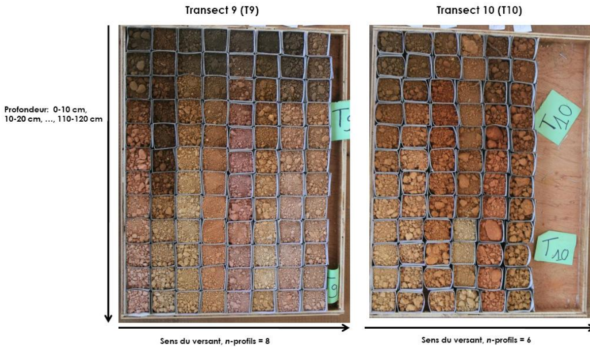
Photos 1.3 Pédocomparateurs issus des prospections sur les transects n° 9 (gauche) et n° 10 (droite).
