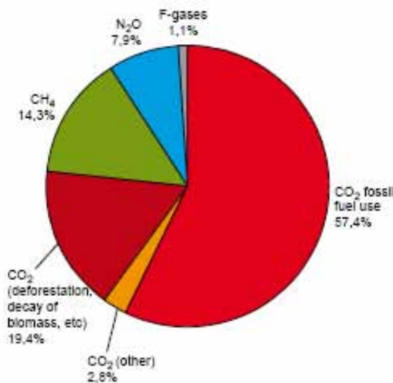
Figure 0.2 Emissions globales de GES anthropiques en 2004 (IPCC, 2007b).
