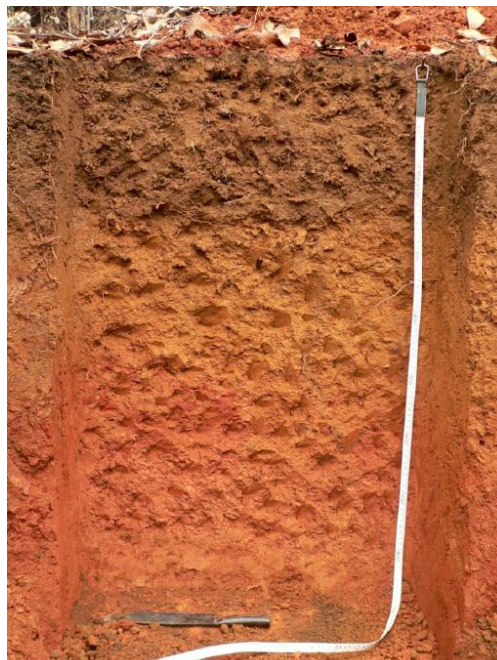
Photo 3.5 Un profil du type de sol (jaune sur rouge) rencontré dans les zones d'étude sur une profondeur de 1m. Photo : Razakamanarivo R.H.
