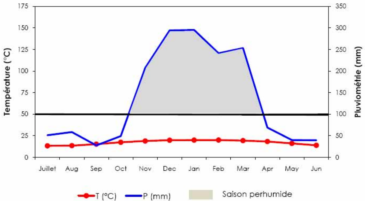
Figure 1.3 Courbes de la température et de la pluviométrie de la région de Manjakandriana (données de 1951 – 1980), Service de la Météorologie, Antananarivo.
