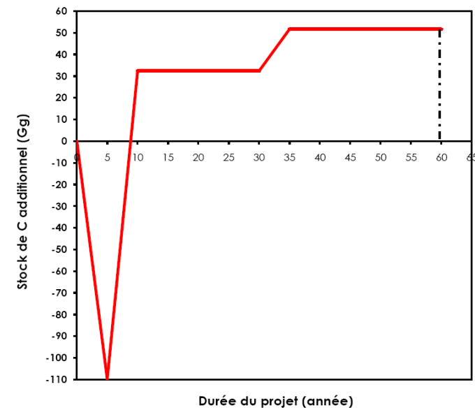
Figure 5.3: Résultats des simulations de prédiction de stocks de C dans la CR de Sadabe : (a) Occupation du u sol à Sadabe et emplacement des parcelles de simulation ; (b) Evolution des stocks de C total (aérien, souterrain, sol) avec la durée du projet/simulation ; (c) Bilan C durant le projet et considérant toutes les parcelles
