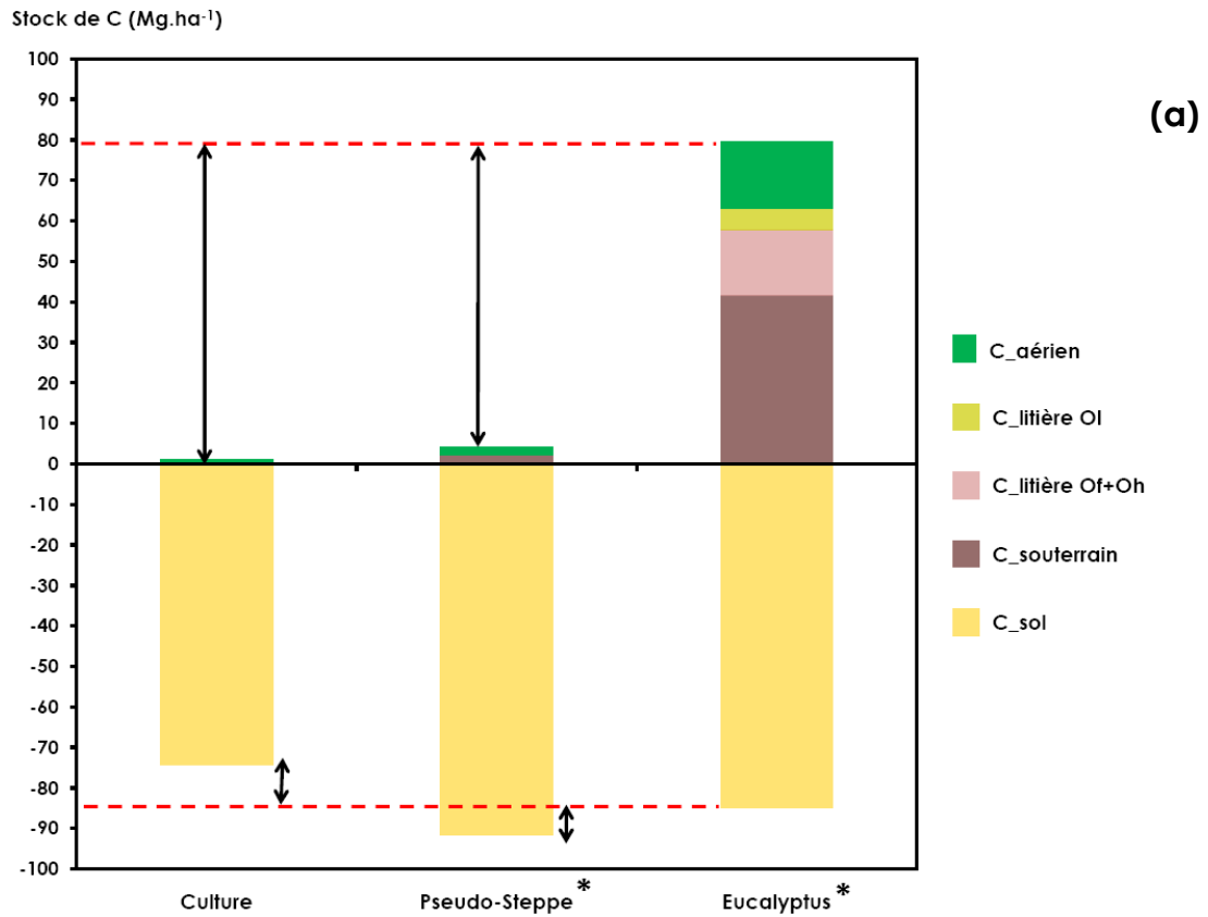
Figure 5-1. Comparaison des stocks de C des différents compartiments entre les trois modes d'usage des terres
