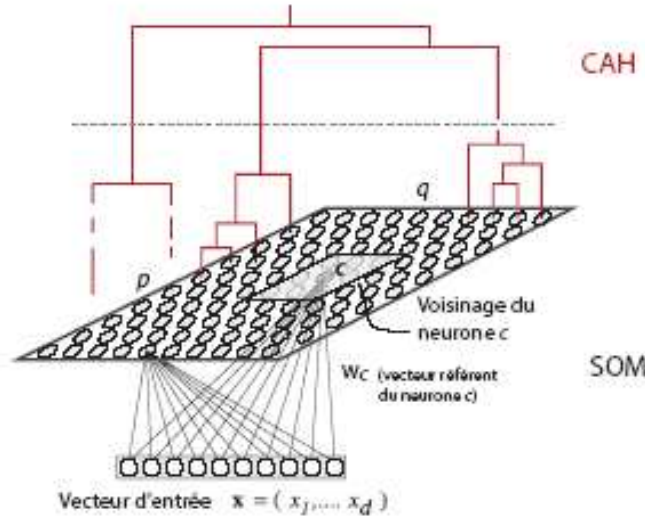
FIGURE 4.6 – Représentation schématique des SOM suivi d'une CAH, d'après Niang et al. (2006) et Leloup (2006).
