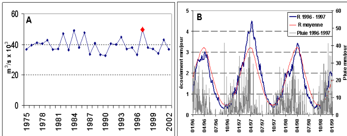
FIGURE 5.7 – A) Crue annuelle à Porto Velho pendant la période 1975–2002 en \text{m}^3/\text{s} \times 10^3 . Le point rouge indique la valeur la plus forte (1997). B) en bleu, écoulement journalier en mm à Porto Velho du 01/01/1996 au 01/01/1999, en rouge, écoulement journalier moyen en mm (1975–2002), en gris, lame d'eau journalière en mm à Porto Velho.
