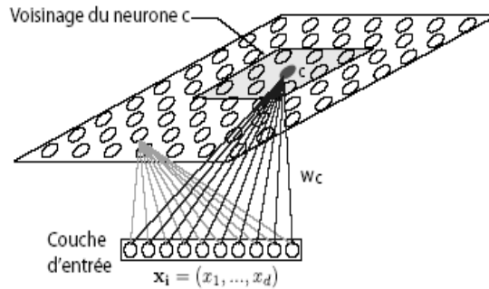
FIGURE 4.1 – Modèle de carte topologique en 2-D, d’après Dreyfus et al. (2002) et Leloup (2006).
