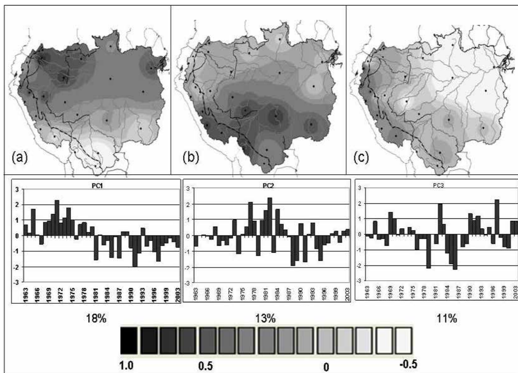
FIGURE 3.32 – Trois principaux modes de variabilité spatio-temporelle, résultant d'une ACP sur les 25 vecteurs pluviométriques régionaux de SON (voir item 2 dans la partie 3.4) dans la période 1963–2003. Le pourcentage de variance associé à chaque mode est indiqué.
