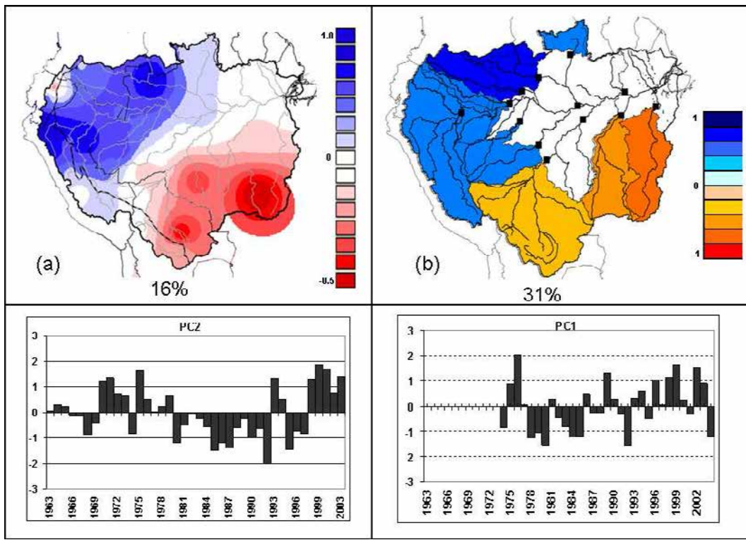
FIGURE 3.34 – (a) Axe 2 de la pluie de MAM pour la période 1963–2003, comme dans la Figure 3.30. (b) Axe 1 des Qmax pour la période 1974–2004, comme dans la Figure 2.8.
