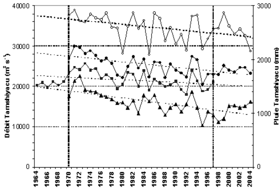
FIGURE A.7 – Rio Amazonas à Tamshiyacu : Variabilité interannuelle des pluies (carrés noirs) et des débits moyens (cercles noirs), minimum (triangles noirs) et maximum (cercles blancs) pour la période 1964–2005.
