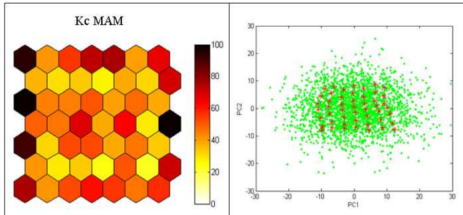
FIGURE 4.11 – Résultat de la méthode neuronale dans la région 10^{\circ}\text{N} - 30^{\circ}\text{S} ; 50 - 80^{\circ}\text{W} . À gauche, la projection de tous les jours de MAM de la période d'étude sur la Kc; à droite, la projection des 49 neurones sur l'espace bidimensionnel des deux composantes principales d'une ACP sur u850 et v850.
