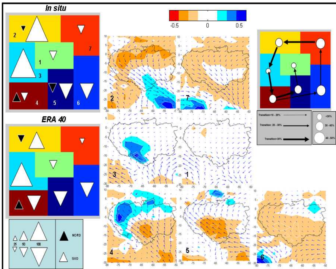
FIGURE 4.20 – Comme la Figure 4.16, mais pour JJA.
