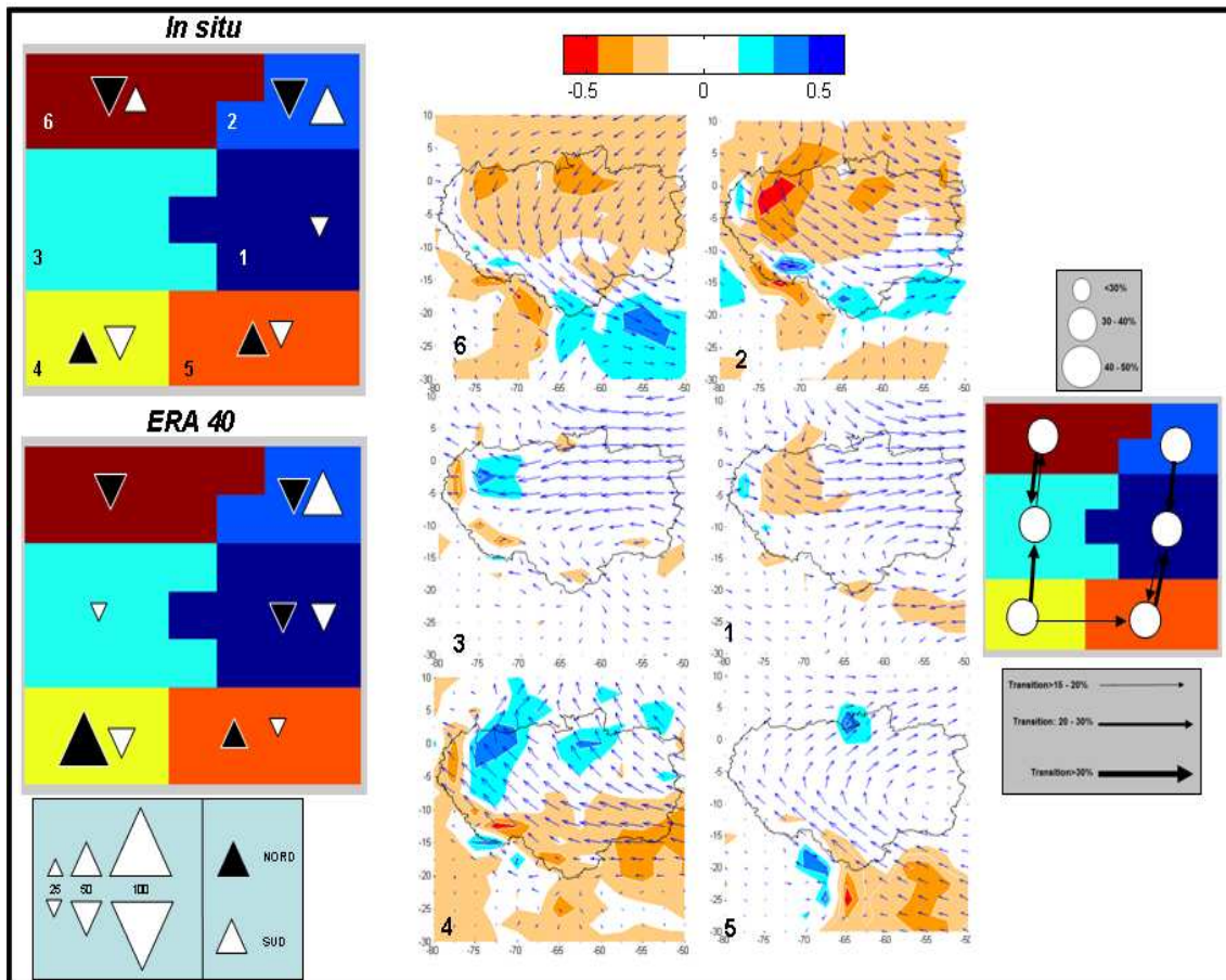
FIGURE 4.26 – Comme la Figure 16, mais pour DJF.
