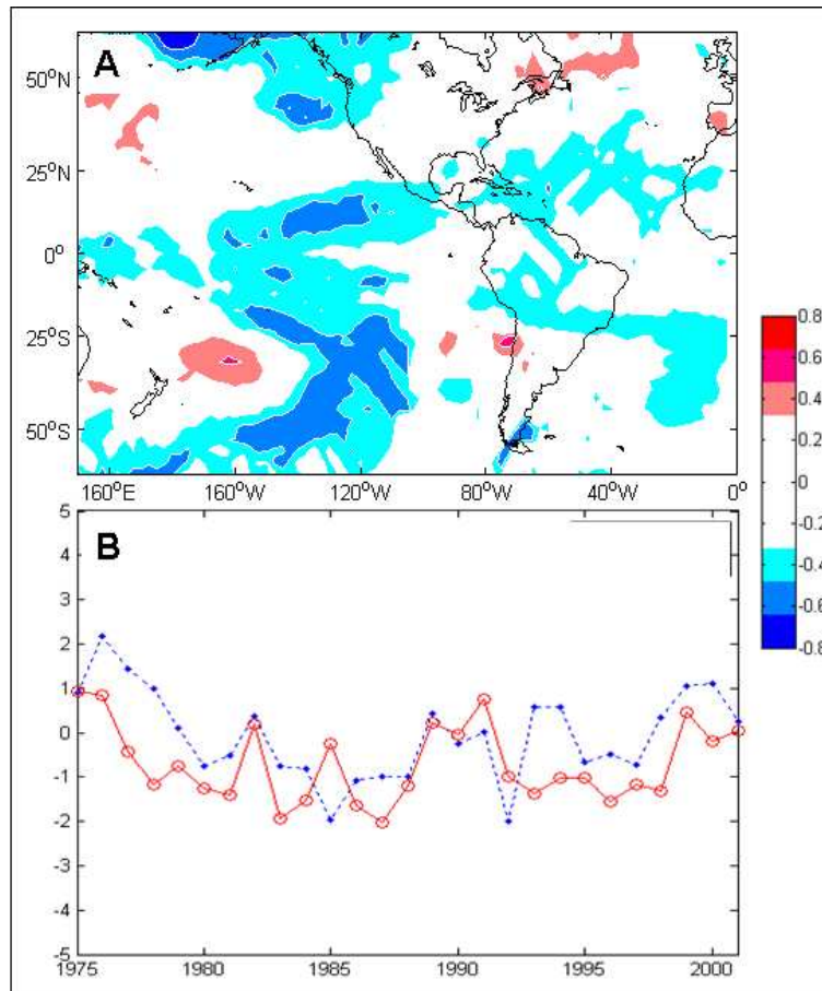
FIGURE 3.44 – A) corrélation entre la SST et la pluie du nord-ouest du BA en MAM (65-80°W ; 5°N-5°S). B) Séries temporelles des anomalies de pluie dans le nord-ouest (ligne bleu ; 65-80°W ; 5°N-5°S) et de la PDO (multipliée par -1, ligne rouge).
