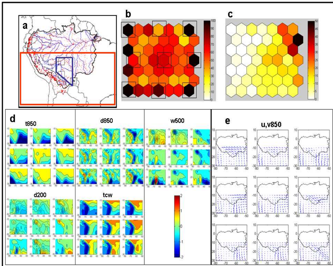
FIGURE 4.9 – Application de la méthode neuronale sur la sous région sud du BA. a) Le cadre rouge définit la région d’analyse dans cette étape du travail. b) projection de tous les jours sur la Kc. c) projection du pourcentage des jours pluvieux sur la Kc. d) conditions moyennes des variables atmosphériques des jours qui se projettent sur les neurones extrêmes (signalés en b). e) Le vecteur vent à 850hPa calculé pour chaque neurone montré en b).
