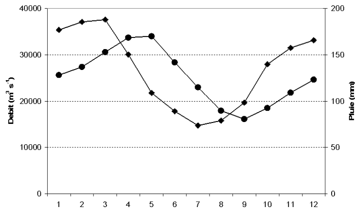
FIGURE A.5 – Cycle annuel moyen des débits (cercles noirs) et des précipitations (carrés noirs) à Tamshiyacu (Rio Amazonas–Pérou)
