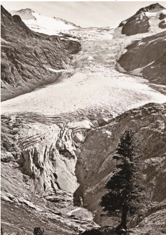
Photographies du Triftgletscher, dans le massif du Dammastock (Alpes suisses) : vers le milieu du XIX e siècle (à gauche) : il y a une dizaine d'années (en bas) : tout récemment en 2002 (à droite).
