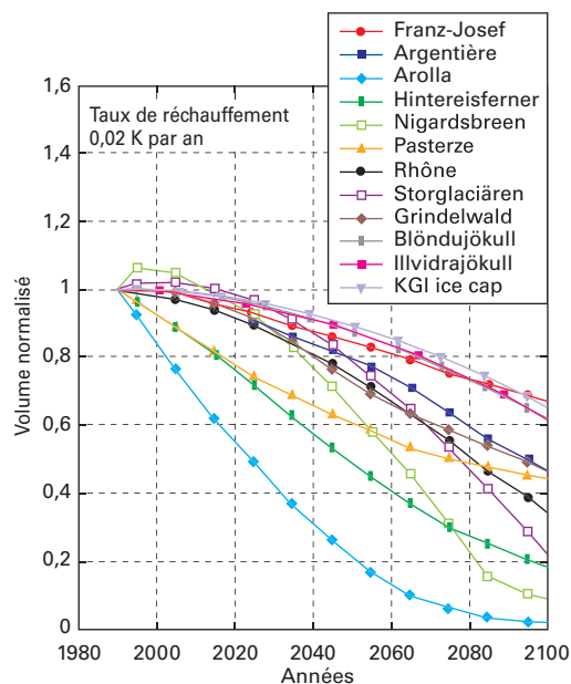
Figure 69 Résultats des simulations EISMINT réalisées avec un taux de réchauffement de 0,02 K par an à partir de 1990 pour les glaciers présentés dans la figure précédente, auxquels ont été rajoutés Blöndujökull, Illvidrajökull (Islande) et KGI Ice cap (Antarctique). Les courbes donnent l'évolution des volumes des glaciers normalisés par rapport à ceux de 1990.
