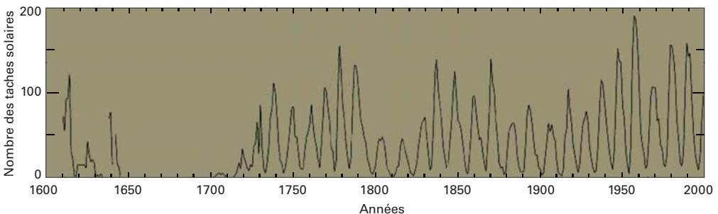
Figure 16 Cycle des taches solaires observées depuis 1600. Les périodes de faible activité coïncident avec les époques réputées pour avoir été froides ou fraîches, 1650-1710 (minimum de Maunder), 1800-1830 (minimum de Dalton), tournant des XIX e -XX e siècles (minimum de 1900), années 1970.
