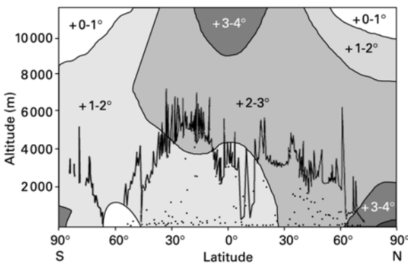
Figure 61 Zones s'étendant du sud au nord des Amériques qui pourraient connaître la même hausse des températures dans le cas où les teneurs en CO 2 de l'atmosphère viendraient à doubler. Les plus fortes hausses à basse altitude (moins de 2 000 m) sont attendues au nord du 30° N, tandis que, sous les tropiques, elles devraient se produire au-dessus de 4 000 m. Trait noir : altimétrie. Points noirs : stations météorologiques existantes. La rareté de ces stations à haute altitude dans la zone intertropicale souligne l'importance des glaciers comme indicateurs du climat.
