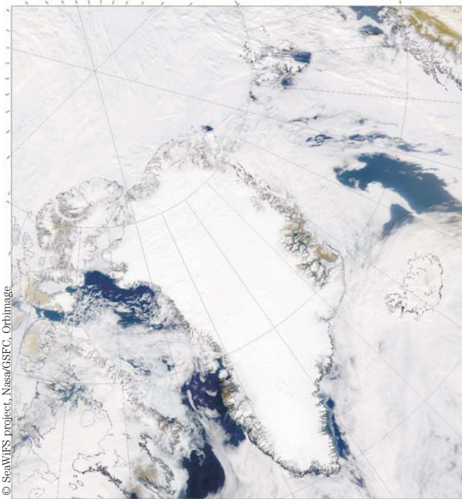
Le Groenland, d'après une image satellitaire prise par SeaWiFS en juillet 2000.
