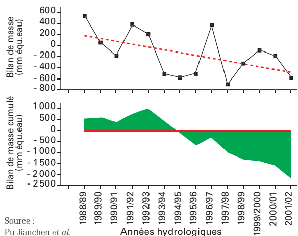
Figure 31 Bilan de masse cumulé du glacier du Xiao Dongkemadi (33° 04' N, 92° 05' E), dans les monts Tanggula au centre du Tibet entre 1988-1989 et 2001-2002. Ce glacier, de 1,7 km 2 et de 2,8 km de long, s'étend entre 5 926 m et 5 380 m. Il est suivi par la Chinese Academy of Sciences à Lanzhou.
