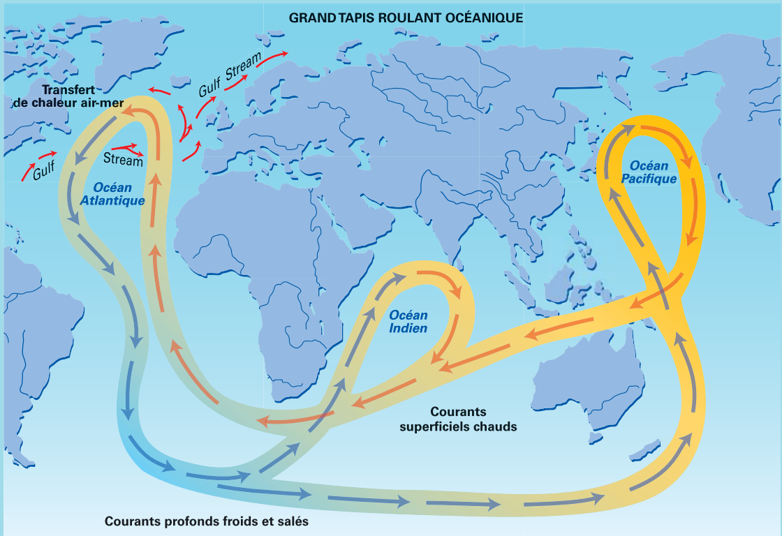
Figure 6 Schéma simplifié de la circulation océanique profonde.
