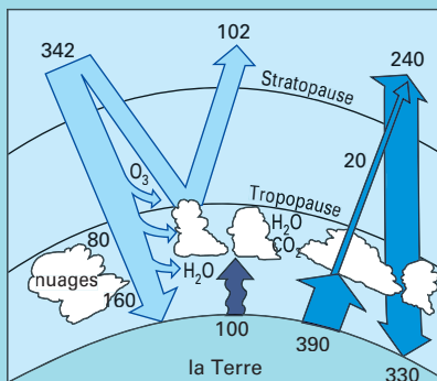
Figure 46 Bilan énergétique moyen de la surface de la terre en W/m^2 . Les arcs de cercle successifs de bas en haut représentent la surface de la Terre, la tropopause (sommet de la troposphère) et la stratopause (sommet de la stratosphère), respectivement.
