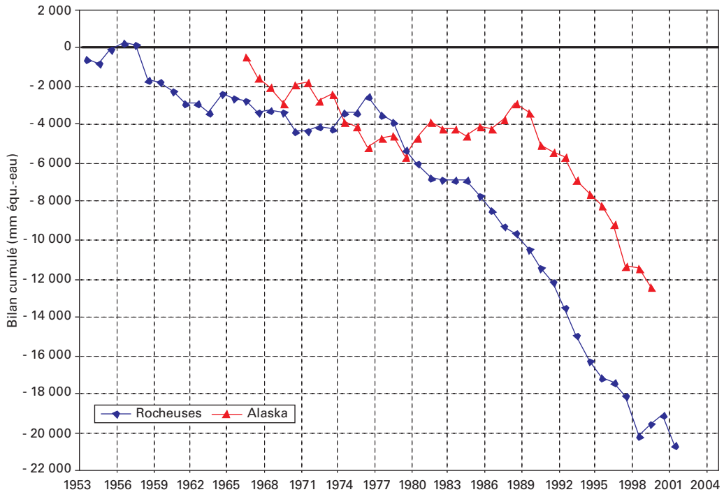
Figure 26 Bilans de masse moyens de deux glaciers d'Alaska (Gulkana, Wolverine) et de huit glaciers des Rocheuses, au sens large, avec extension aux chaînes côtières du Pacifique (Blue, Helm, Lemon-Creek, Peyto, Place, Sentinel, South Cascade). Augmentation des pertes au sud dès 1976, alors qu'elle se manifeste plus tard, pendant la décennie 1990, sur les glaciers surveillés d'Alaska. Depuis, les déficits se creusent à un rythme à peu près similaire sur toute l'Amérique du Nord. L'Arctique n'est pas considéré ici.
