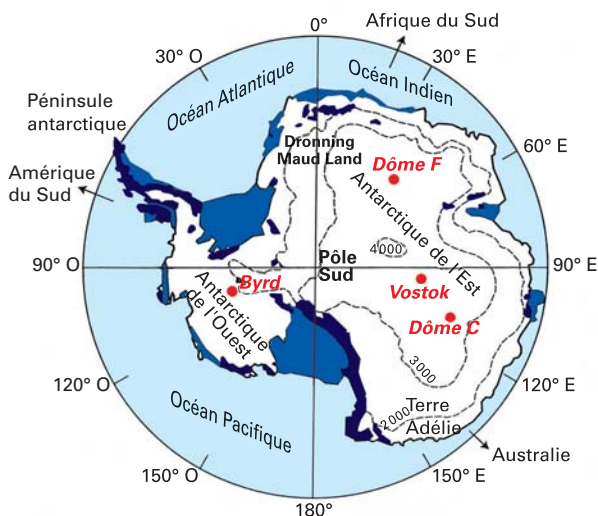
Figure 48 L'Antarctique et ses diverses régions. En rouge : situation des grands forages.
