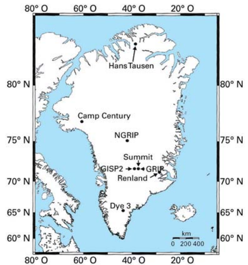
Figure 4 Le Groenland, avec les sites de forages principaux.
