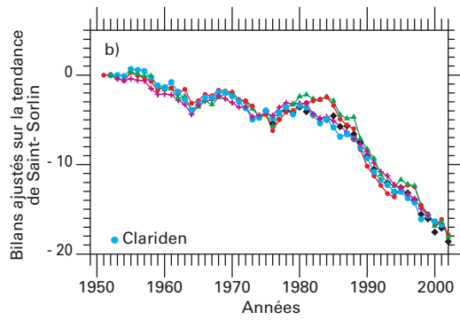
Figure 22 Bilans de masse cumulés de cinq glaciers des Alpes françaises, autrichiennes et suisses au cours des cinquante dernières années (à gauche). Lorsque l'on retire à chacune des valeurs de bilans annuels la moyenne des cinquante dernières années, on obtient alors (à droite) un signal remarquablement commun pour l'ensemble de ces glaciers (les plus éloignés sont à 400 km de distance). Ce signal commun traduit les variations climatiques à l'échelle des Alpes. Les petits triangles représentent les observations directes de terrain, à partir des carottages et des balises d'ablation ; les triangles larges représentent des résultats obtenus avec la photogrammétrie.
