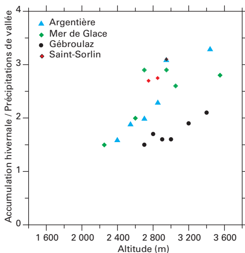
Figure 45 Rapport entre l'accumulation hivernale observée sur le glacier et les précipitations hivernales mesurées dans les stations des vallées voisines en fonction de l'altitude. Comme on le voit, ce rapport peut atteindre des valeurs supérieures à 3.
