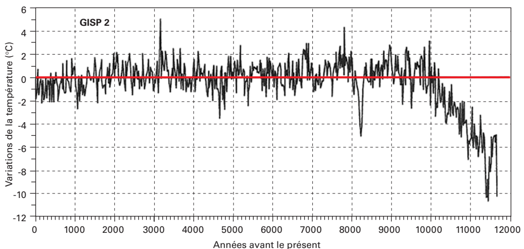
Figure 7 Variations de la température du Groenland par rapport à l'actuelle, reconstituées à partir des isotopes de la glace et des paléotempératures au trou de forage du site GISP2.
