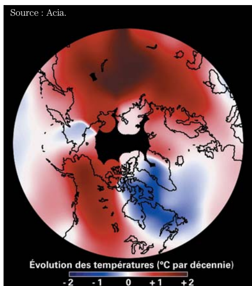
Figure 57 Augmentation des températures hivernales dans l'Arctique de 1966 à 1995. En blanc et bleu, les zones où la température est restée égale ou a baissé ; en rouge, les zones où elle a augmenté. L'échelle du bas donne les valeurs correspondant aux couleurs.
