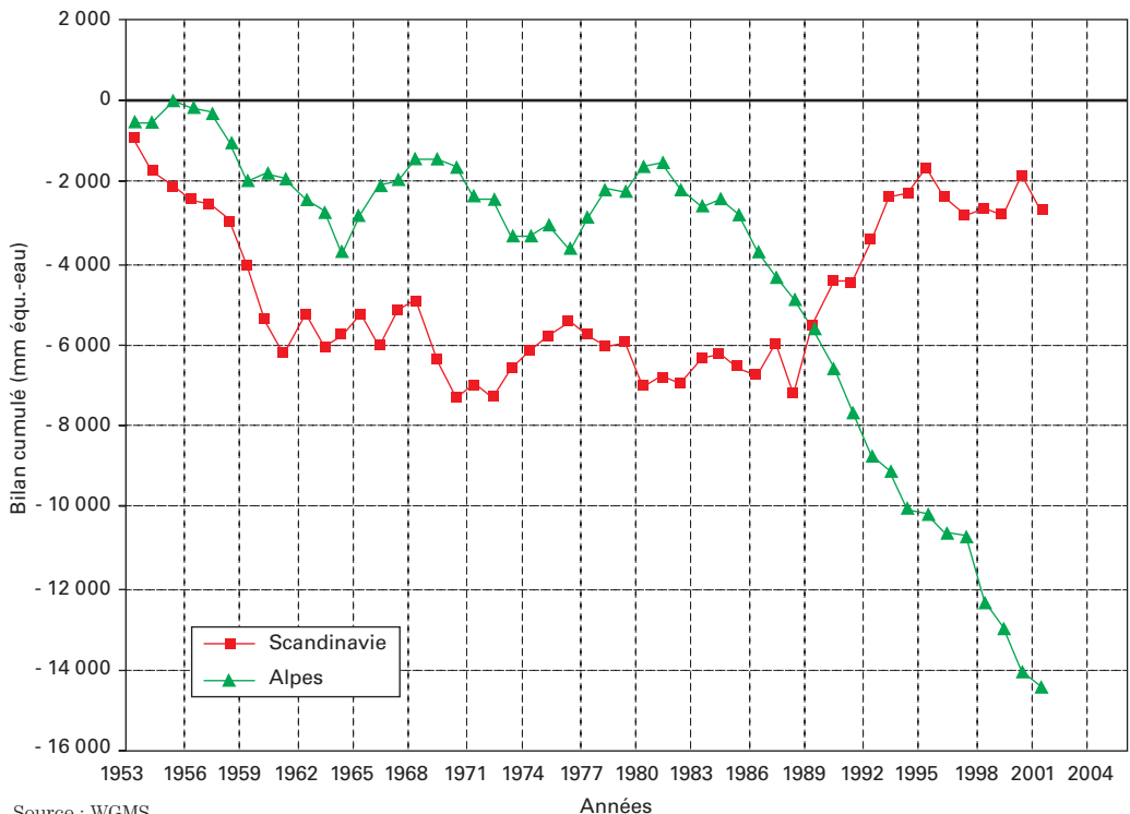
Figure 25 Bilans de masse moyens de neuf glaciers scandinaves (en rouge) et de quatorze glaciers des Alpes (en vert). En rouge : Ålfotbreen, Engabreen, Gråsübreen, Hardangerjoekulen, Hellstugubreen, Nigardsbreen, Rabots, Storbreen, Storglaciären. En vert : Aletsch, Careser, Gries, Hintereis, Jamtal, Kesselwand, Limmern, Plattalva, Saint-Sorlin, Sarennes, Silvretta, Sonnblick, Vergagt, Wurten. Les bilans sont présentés sous forme cumulée.
