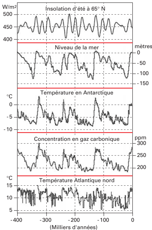
Figure 2 Variation de l'insolation d'été à 65° N (en W/m 2 ), du niveau de la mer, de la température en Antarctique, de la concentration de gaz carbonique (CO 2 ) et de la température en Atlantique nord durant les 400 000 dernières années. Sur cette période, on observe nettement 4 périodes glaciaires et 5 interglaciaires, avec une périodicité proche de 100 000 ans. À noter que les taux maximum de concentration de CO 2 dans l'atmosphère pendant les périodes interglaciaires sont typiquement compris entre un peu plus de 250 ppm et un peu moins de 300 ppm. Les réchauffements marquant les périodes interglaciaires sont asymétriques, avec une phase de réchauffement brutal suivie d'une phase de dégradation plus lente des températures.
