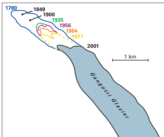
Figure 30 Positionnement des fronts successifs du glacier de Gangotri (Himalaya du Garhwal) depuis 1780.
