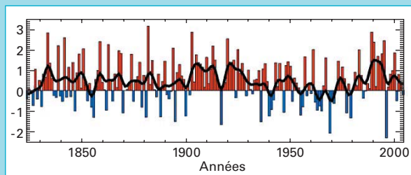
Figure 53 L'indice d'oscillation Nord-Atlantique de 1823 à 2004. Le NAO index est défini comme la différence normalisée entre les hautes pressions subtropicales (Lisbonne, Portugal) et les basses pressions subpolaires (Stykkisholmur, Islande) pendant l'hiver (de décembre à mars). La courbe présente les données lissées.
