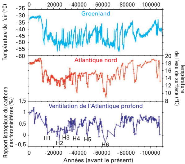
Figure 5 Température de l'air au Groenland (en °C) d'après la composition isotopique de la glace (haut). Température (en °C) des eaux de surface de l'Atlantique nord d'après des molécules spécifiques du phytoplancton conservées dans les sédiments prélevés par des carottes océaniques au large du Portugal (milieu). La ventilation des eaux profondes de l'Atlantique (bas) est reconstituée à partir des isotopes du carbone provenant de micro-organismes marins prélevés dans ces carottes. Les événements de Heinrich (H1 à H6) correspondent à des refroidissements brutaux.
