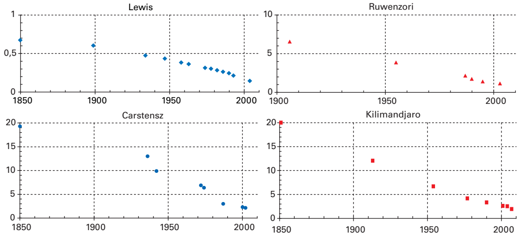
Figure 32 Évolution des surfaces (en km 2 ) des glaciers Lewis (Mont Kenya) et au Carstensz (Papouasie-Nouvelle-Guinée).
