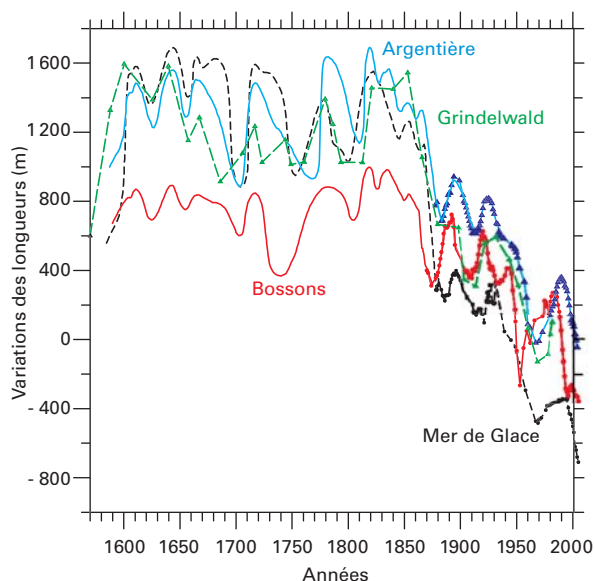
Figure 10 Fluctuations de longueur de quatre glaciers dans les Alpes : Mer de Glace, Argentièrre, Bossons, Grindelwald. L'origine 0, dans l'échelle de variations des longueurs, est arbitraire. Noter comment le glacier des Bossons anticipe de quelques années les variations de ses voisins, Mer de Glace et Argentièrre.
