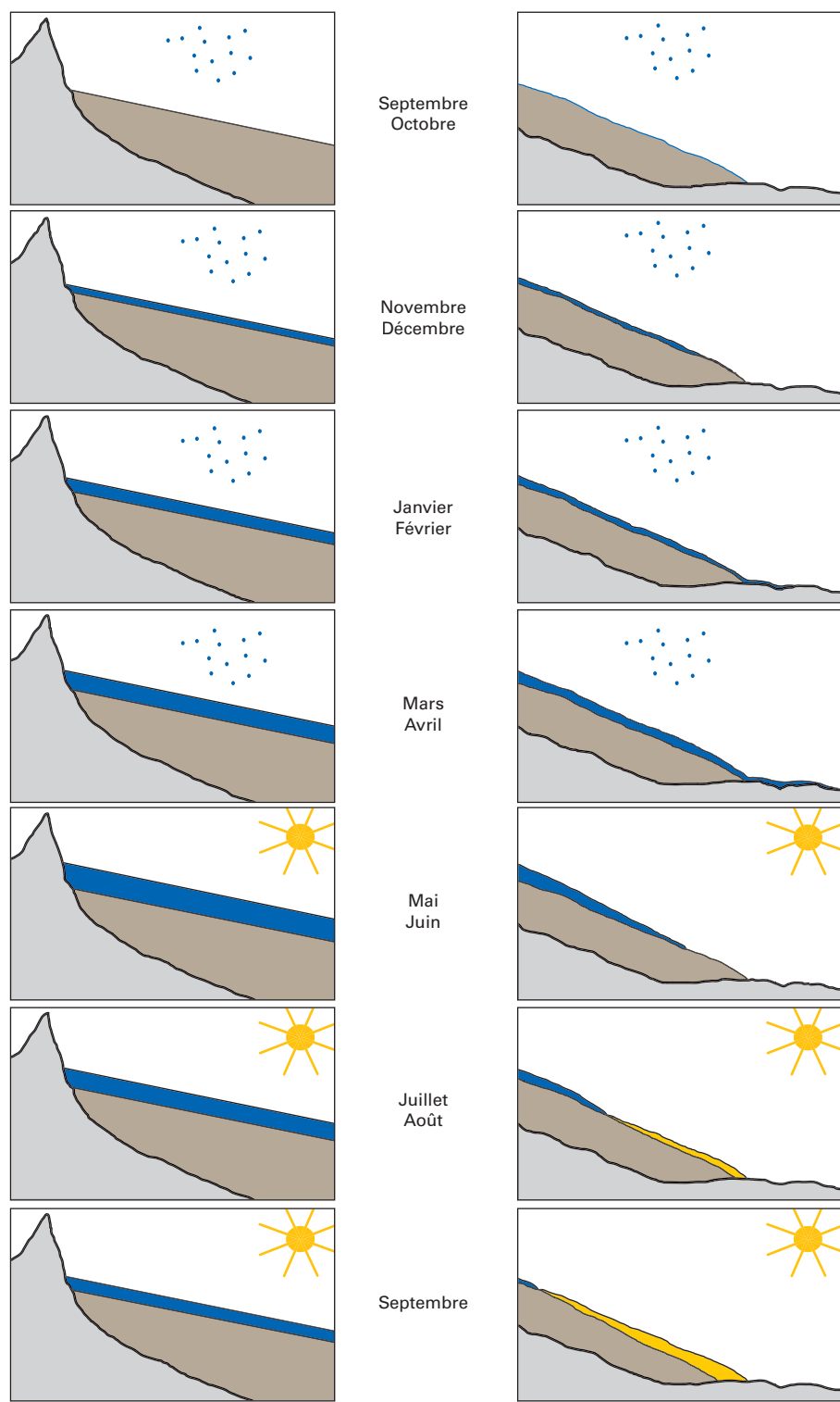
Figure 43 Schéma simplifié de l'évolution des bilans de masse de surface pendant une saison hydrologique dans les Alpes, à gauche dans la zone haute d'un glacier vers 3 500 m d'altitude, à droite au front d'un glacier vers 2 500 m. En bleu, l'accumulation de neige, en jaune l'ablation de glace. Le soleil indique les périodes d'ablation, les autres situations sont des périodes d'accumulation. Il s'agit là d'une année moyenne.
