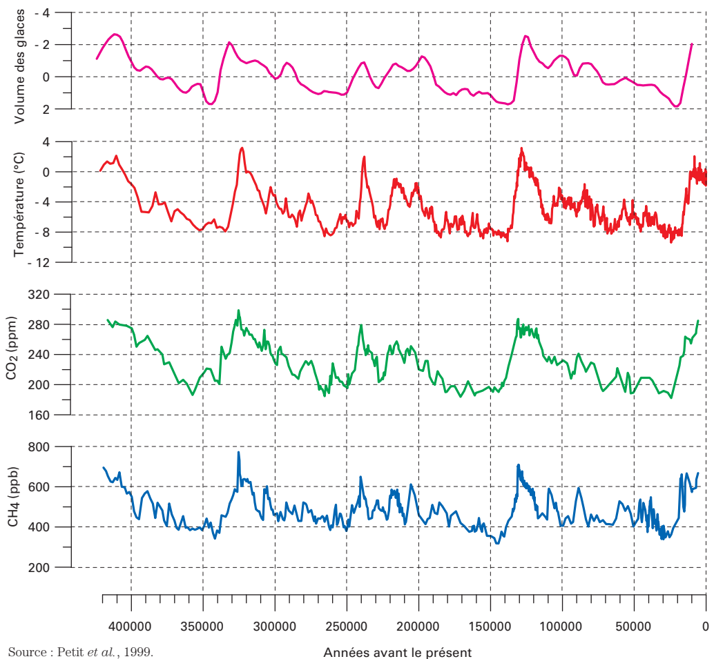
Figure 1 Les cycles glaciaires/interglaciaires depuis 420 000 ans selon le carottage de Vostok (Antarctique). Volume des glaces ; température ; gaz carbonique ; méthane.
