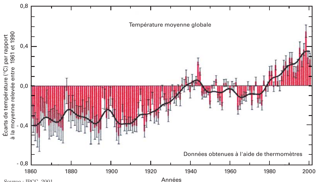
Figure 18 Anomalies relevées dans les températures annuelles à la surface de la Terre de 1861 à 2000. Ces températures combinent des données provenant de la surface des continents et des océans et sont représentées en écarts par rapport à la moyenne de la période 1961-1990. Les barres d'incertitude représentent deux écarts-types de la température annuelle.
