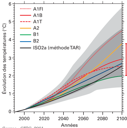
Figure 60 Simulations des températures obtenues par différents modèles selon divers scénarios d'émission de gaz à effet de serre. Les scénarios dits « modérés » sont compris entre 2,0 °C et 3,5 °C (trait rouge vertical). Les scénarios A1 et B1 envisagent des croissances économiques rapides et globales, avec un recours plus (A1) ou moins (B1) marqué aux énergies fossiles, tandis que les scénarios A2 et B2 misent sur des mondes plus hétérogènes où la croissance est plus lente et la protection de l'environnement plus (B2) ou moins (A2) mise en pratique.
