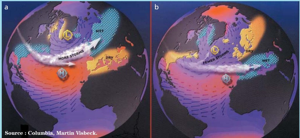
Figure 52 L'oscillation Nord-Atlantique avec les deux phases extrêmes, la phase positive, à gauche, et la phase négative, à droite. En bleu et jaune, les régions anormalement humides et sèche, respectivement, dans les mois d'hiver.
