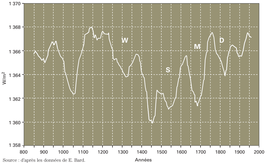
Figure 17 Évolution de l'éclairement solaire, reconstituée à partir de la production de ^{10}\text{Be} observée dans les glaces des forages de l'Antarctique par Bard et al. (2000) depuis 850 apr. J.-C. Les lettres W, S, M, D désignent les minima d'intensité de Wolf, Spörer, Maunder et Dalton, respectivement. La calibration de la courbe de l'irradiance est réalisée selon l'hypothèse d'une baisse de 0,4 % pendant le minimum de Maunder.
