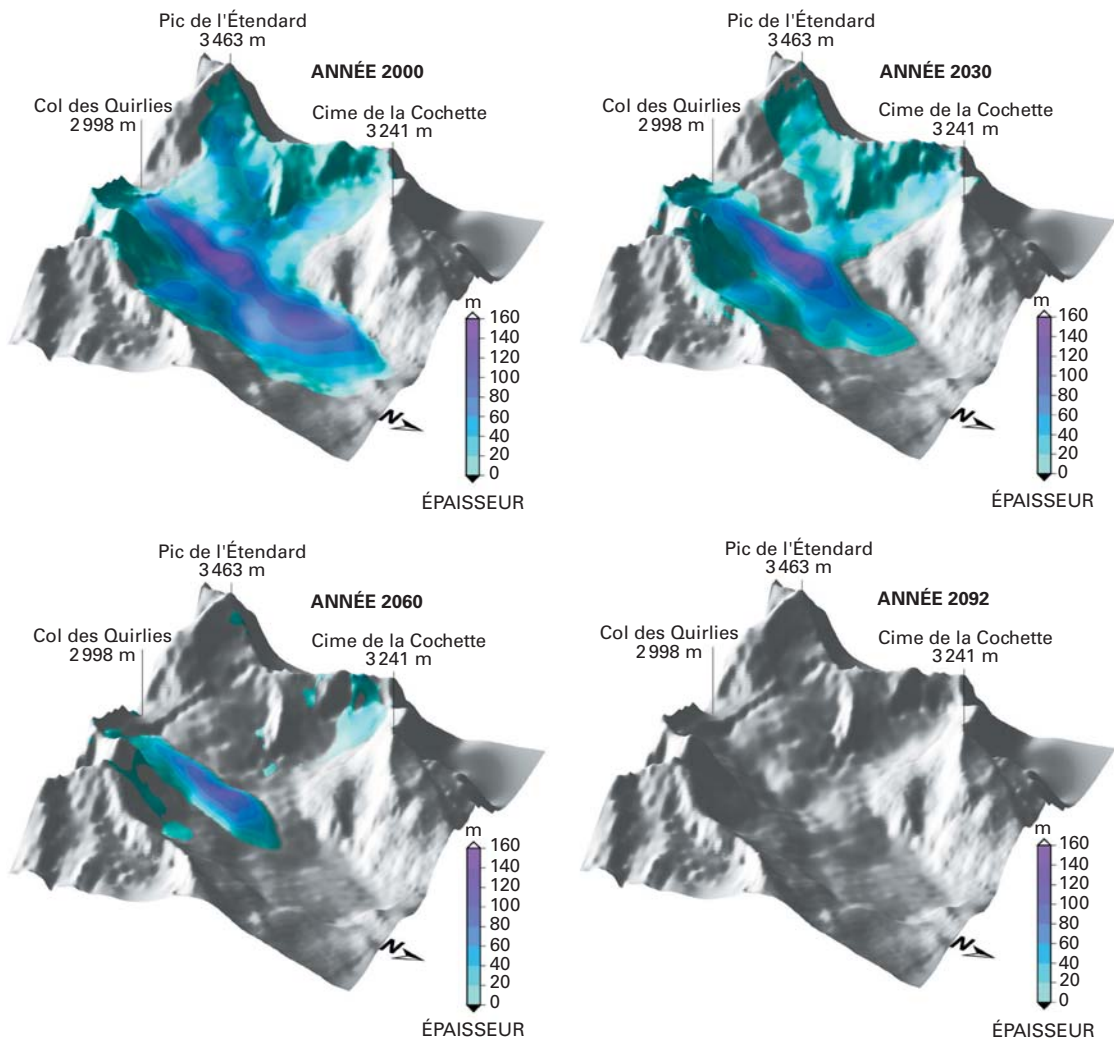
Figure 67 Résultats d'une simulation de l'évolution du glacier de Saint-Sorlin réalisée selon un scénario climatique prévoyant une hausse de 2,0 °C/2,5 °C d'ici la fin du XXI e siècle. De gauche à droite et de haut en bas, formes du glacier prévues en 2000, 2030, 2060 et 2092.
