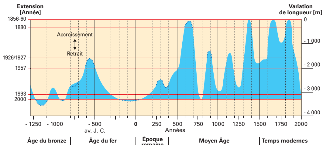
Figure 9 Phases d'avancée et de retrait du grand glacier d'Aletsch depuis 1300 av. J.-C. À droite, variations de longueur avec comme référence le maximum de 1856-1860 (= 0). À gauche, les extensions des années de référence.
