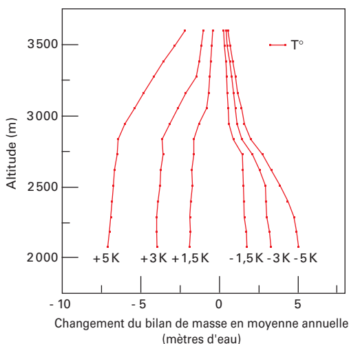
Figure 63 Influence de la température sur le bilan de masse en fonction de l'altitude. Ces calculs ont été réalisés sur un glacier alpin (fictif) exposé au nord avec une pente régulière de 20°. Les changements des bilans de masse ont été calculés suivant différents scénarios climatiques (+1,5 °C, +3 °C, +5 °C) à différentes altitudes. Par exemple, à 2 000 m d'altitude, une augmentation de température de 3 °C impliquerait une diminution du bilan de masse d'environ 4 m d'équivalent eau. Températures en degrés Celsius.
