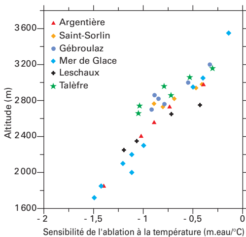
Figure 62 Sensibilité de l'ablation à la température estivale en fonction de l'altitude. Les points représentent la variation de la fonte estivale que l'on peut attendre d'un réchauffement estival de 1 °C. Ainsi, sur le glacier d'Argentière vers 2400 m, un réchauffement d'été de 1 °C ferait monter l'ablation annuelle de 1 m environ.
