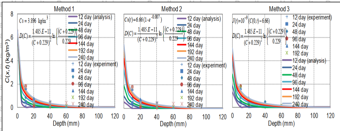
Gambar 2.5 Profil klorida terhadap waktu H-40 dengan 3 metode
