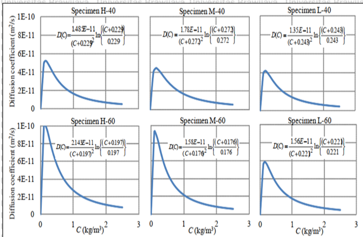
Gambar 2.7 Koefisien difusi terhadap klorida Sumber : Nuralinah, 2012
