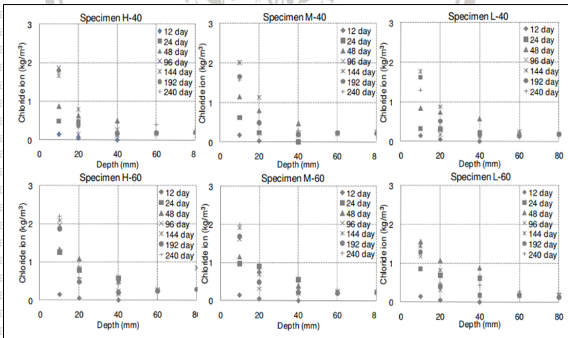
Gambar 2.6 Data kadar klorida terhadap waktu dan kedalaman
