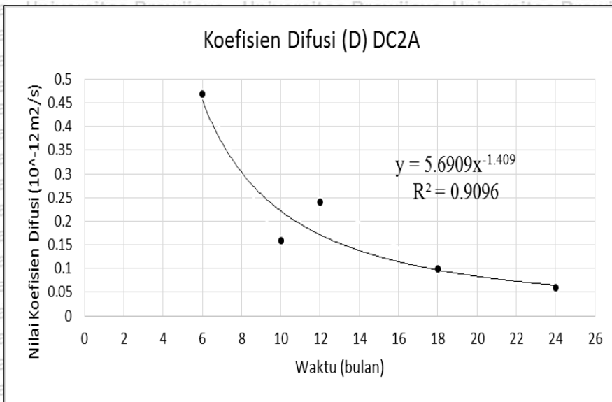
Gambar 4.11 Koefisien difusi klorida DC2A
