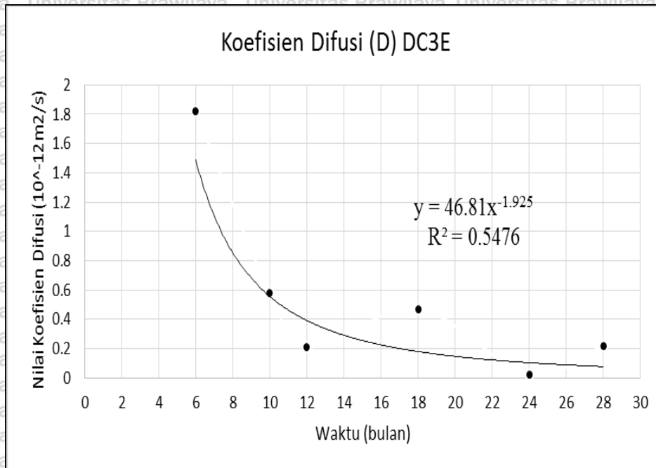
Gambar 4.18 Koefisien difusi klorida DC3E
