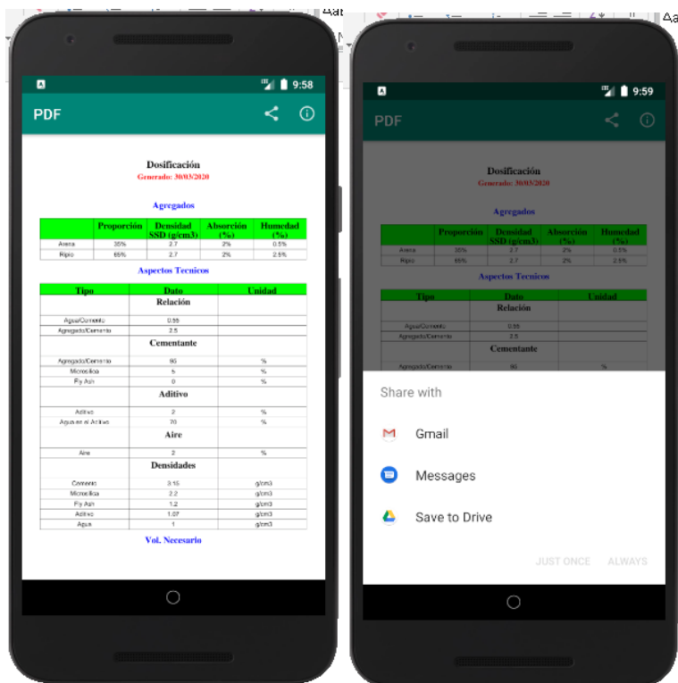
Figura 17. Actividad ViewPDFActivity. Fuente: Android Studio, 2020.
