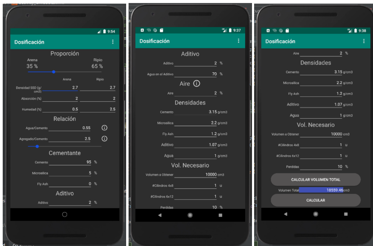
Figura 9. Actividad MainActivity. Fuente: Android Studio, 2020.
