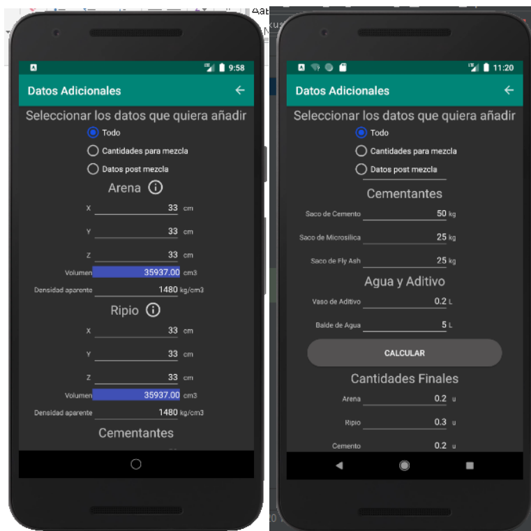
Figura 13. Actividad DatosAdicionales (a). Fuente: Android Studio, 2020.
