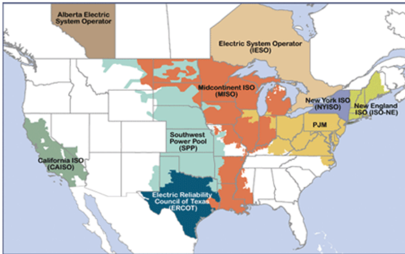
Figure 1: RTO/ISO Map
