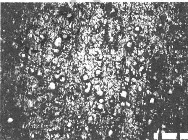
Рис. 3. Микроструктура дюралюминия (продольное сечение) в зависимости от степени деформации: а – Т-Д-прокатка, б – стандартная прокатка (одно деление 10 мкм). \times 2000
