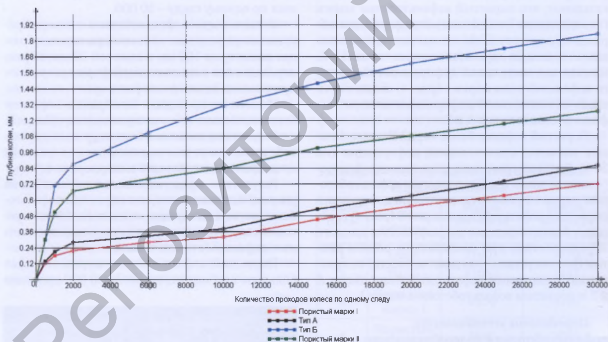
Рисунок 6 – Зависимость глубины колеи от количества проходов колеса
