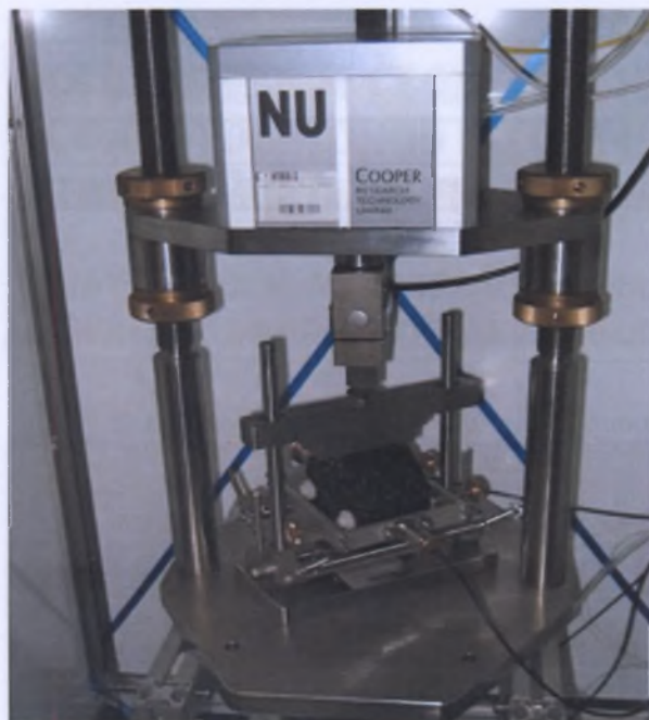
Рисунок 2 – Определение модуля жесткости асфальтобетонного образца на установке «Nottingham»
