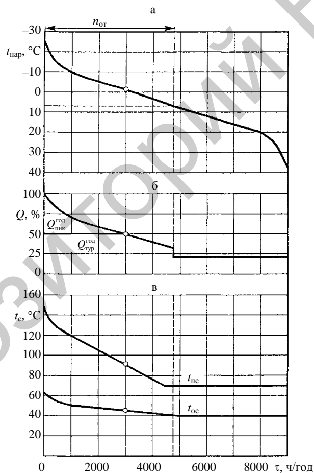
Рис. 2. Типичные годовые графики: а – температура наружного воздуха; б – тепловая нагрузка; в – температура сетевой воды; Q_{тур}^{год} , Q_{пик}^{год} – годовой отпуск теплоты от турбины и пикового источника; t_{пс} , t_{ос} – температура прямой и обратной сетевой воды; n – годовая продолжительность; n_{от} – отопительный период; о – расчетная предельная точка отборов пара турбины ( \alpha_{тэц}^{час} = 0,5 , где \alpha_{тэц}^{час} – коэффициент часовой теплофикации)
