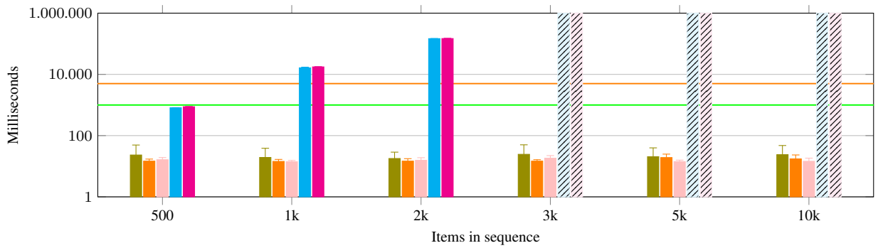
(b) Virtuoso
