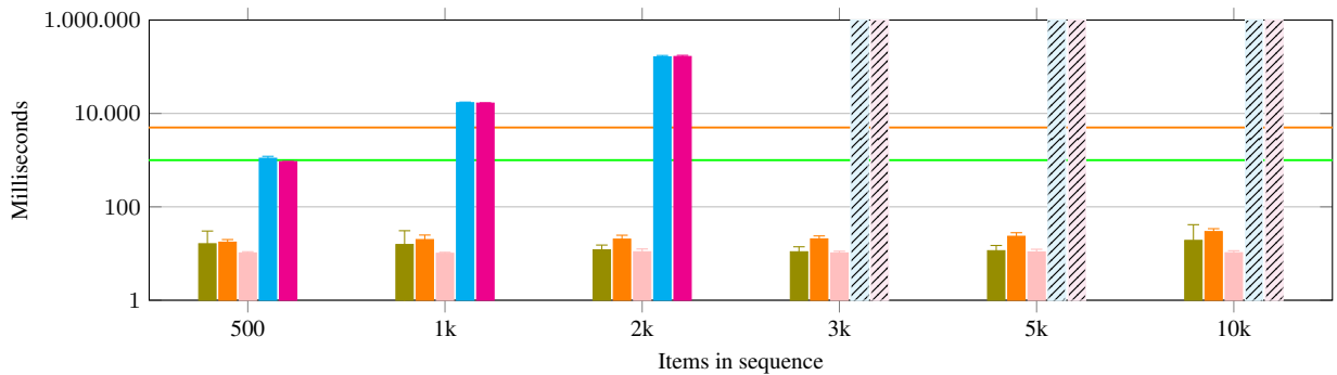
(b) Virtuoso
