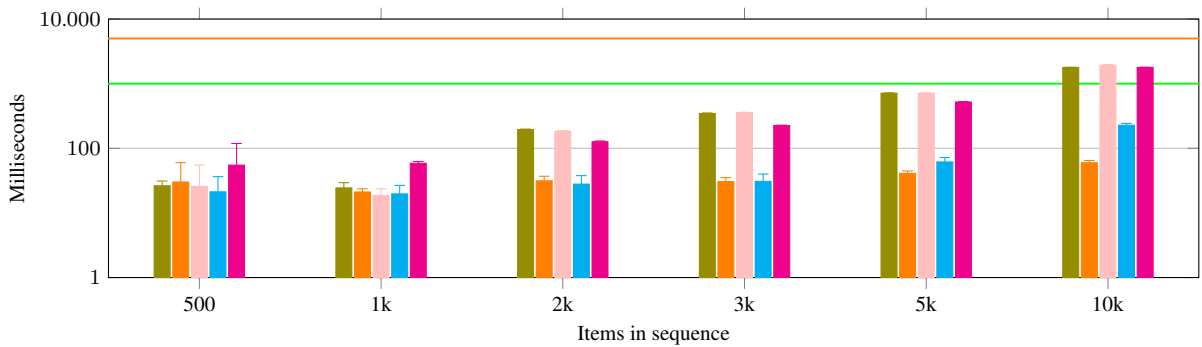
(b) Virtuoso
