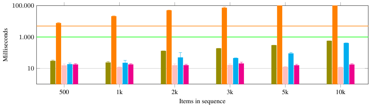
(b) Virtuoso
