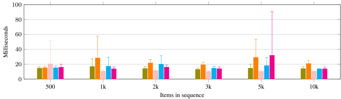
(b) Virtuoso
