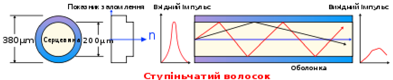
Рис. 1.3 Багатомодове волокно
