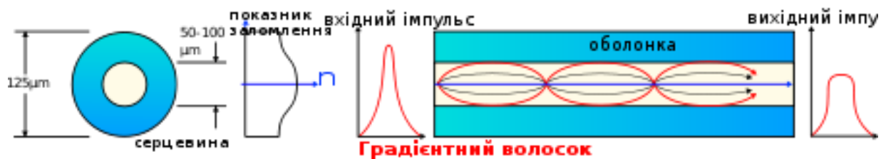
Рис. 1.4 Градієнтне волокно
