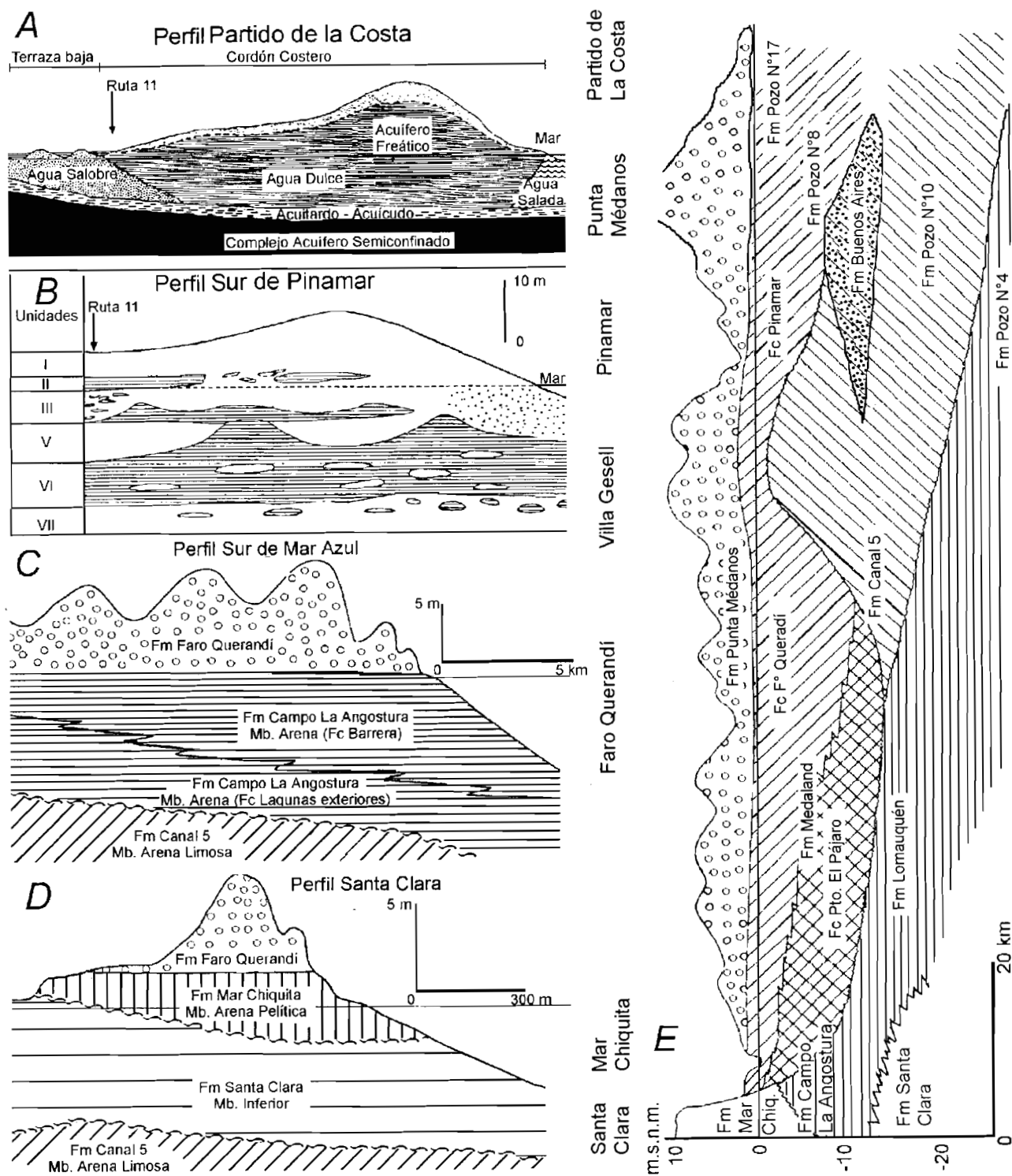
Figura 3. Modelo hidrogeológico para: A- Partido de la Costa (CFI, 1990), B- Sur de Pinamar (González Arzac et al., 1992), C- Sur de Mar Azul (Fasano, 1991) y D- Santa Clara (Fasano, 1991); relacionados a F- Perfil Geológico (Sur-Norte) entre Mar Chiquita y Partido de la Costa (modificado de Parker y Violante, 1989).
