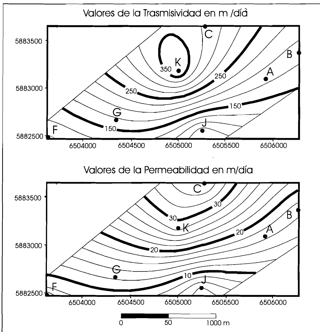
Figura 6. Datos de Trasmisividad ( m^2/día ) y Permeabilidad ( m/día ) integrados.
