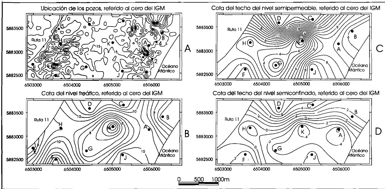
Figura 2. Ubicación de los pozos en el modelo digital de terreno (A) y planos del nivel freático (B), techo del semipermeable (C) y techo del semiconfinado (D). Todos referidos a la cota del IGM.
