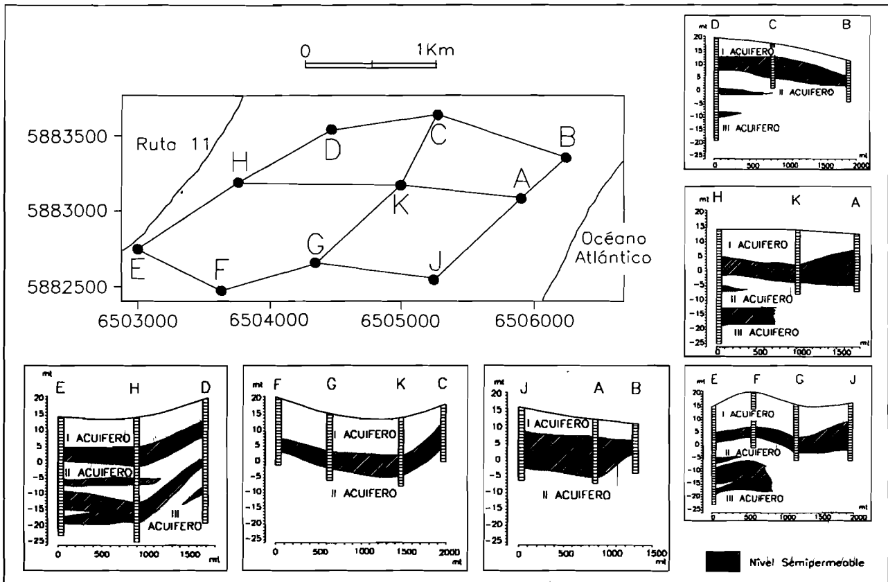
Figura 5. Esquema hidrodinámico al sur de Cariló.
