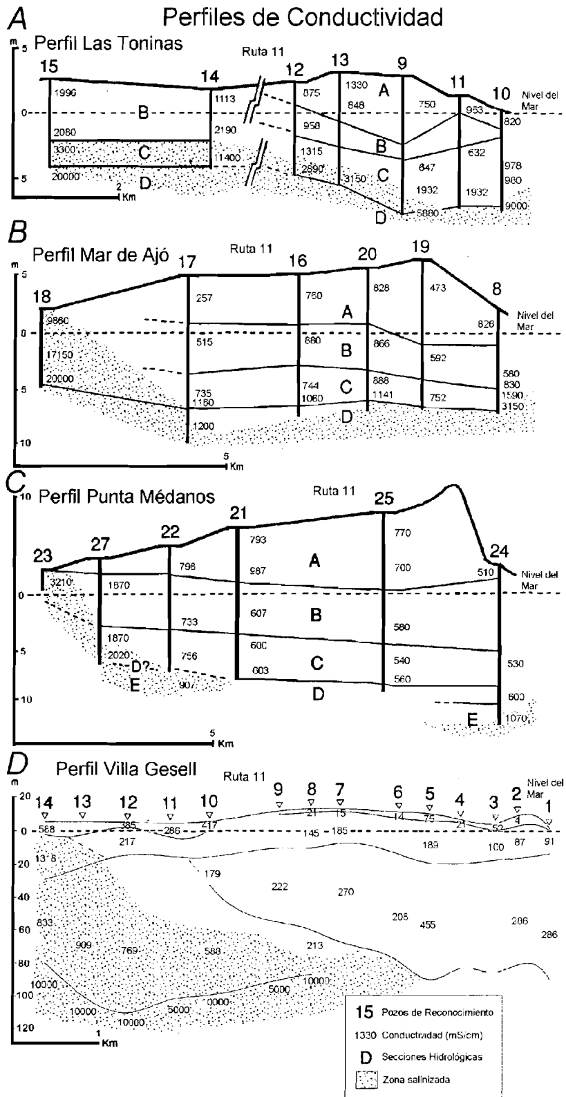
Figura 4. Perfiles de conductividad en las localidades de A- Las Toninas, B- Mar de Ajó, C- Punta Médanos (modificado de CFI, 1990) y D- Villa Gesell (modificado de Hurtado et al. , 1987).
