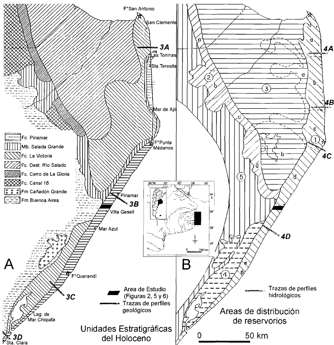
Figura 1. A- Mapa de ubicación. Unidades estratigráficas del Holoceno y trazas de los perfiles geológicos de la Figura 4 (modificado de Parker y Violante, 1989). B- Áreas de distribución de reservorios y trazas de los perfiles hidrológicos de la Figura 5 (modificado de Parker y Violante, 1989).
