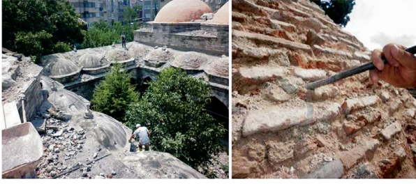
Fotoğraf 20. İmaret kubbeleri: Kurşun taklidi çimento şap ve çimento harçlı derz raspası yapılırken, 2011 (Ebru Sünnetçi)
