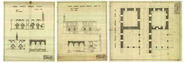
Şekil 5. Sıbyan Mektebi rölovesi, 1967 (Vakıflar Arşivi)
