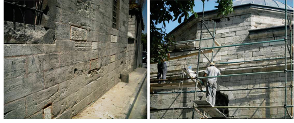
Fotoğraf 24. Taş çürütme sonrasında sağlamlaştırma işlemi, 2011 (Ebru Sünnetçi)
