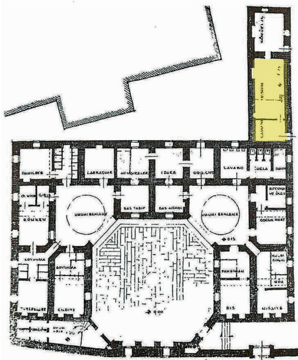
Şekil 4. Darüşifâ planı, Orhan Bolak rölovesi, 1950 (Taşkıran 1972: 253)
