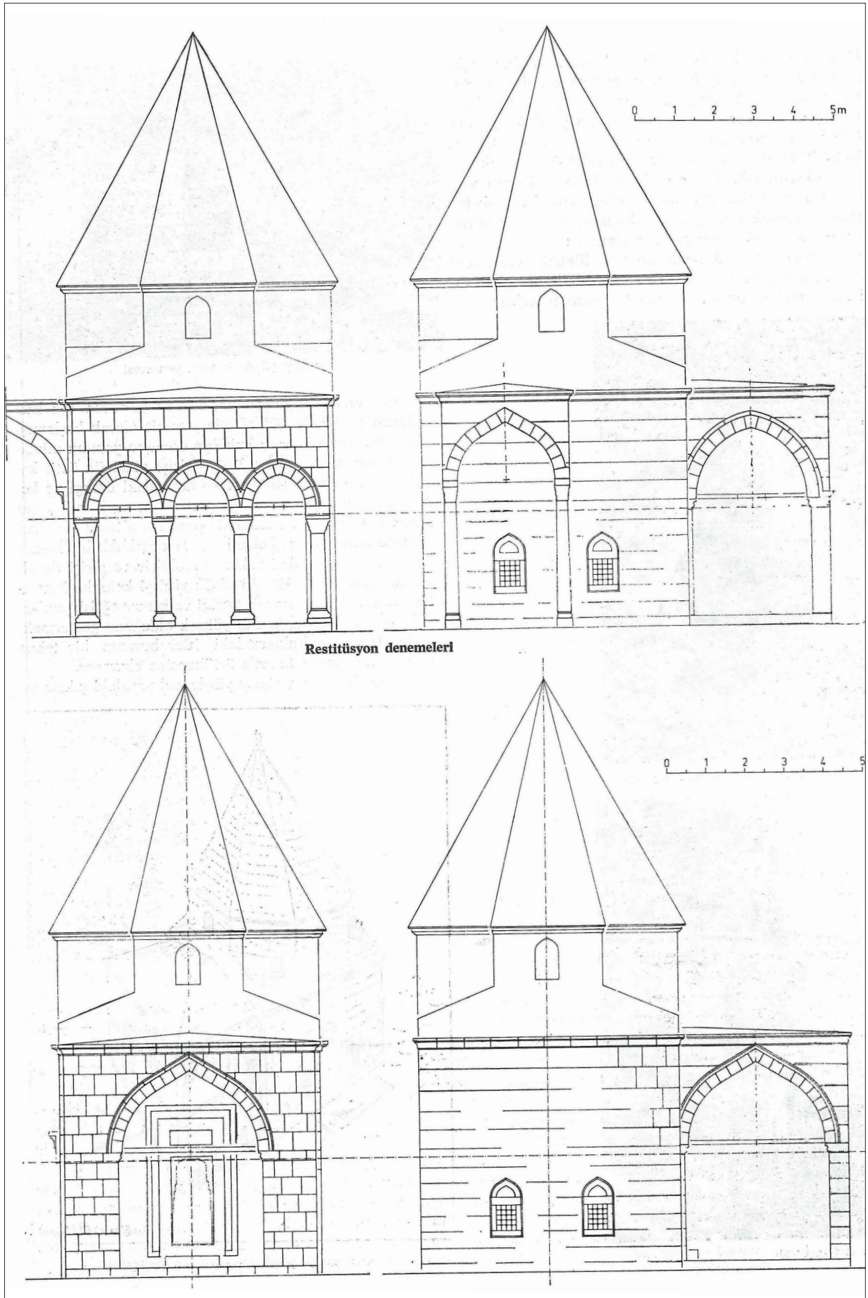
Şekil 11. Ankara Polatlı Hacı Tuğrul Türbesi Restitüsyon denemeleri (Kaynak: Tuncer 1991: 28)
