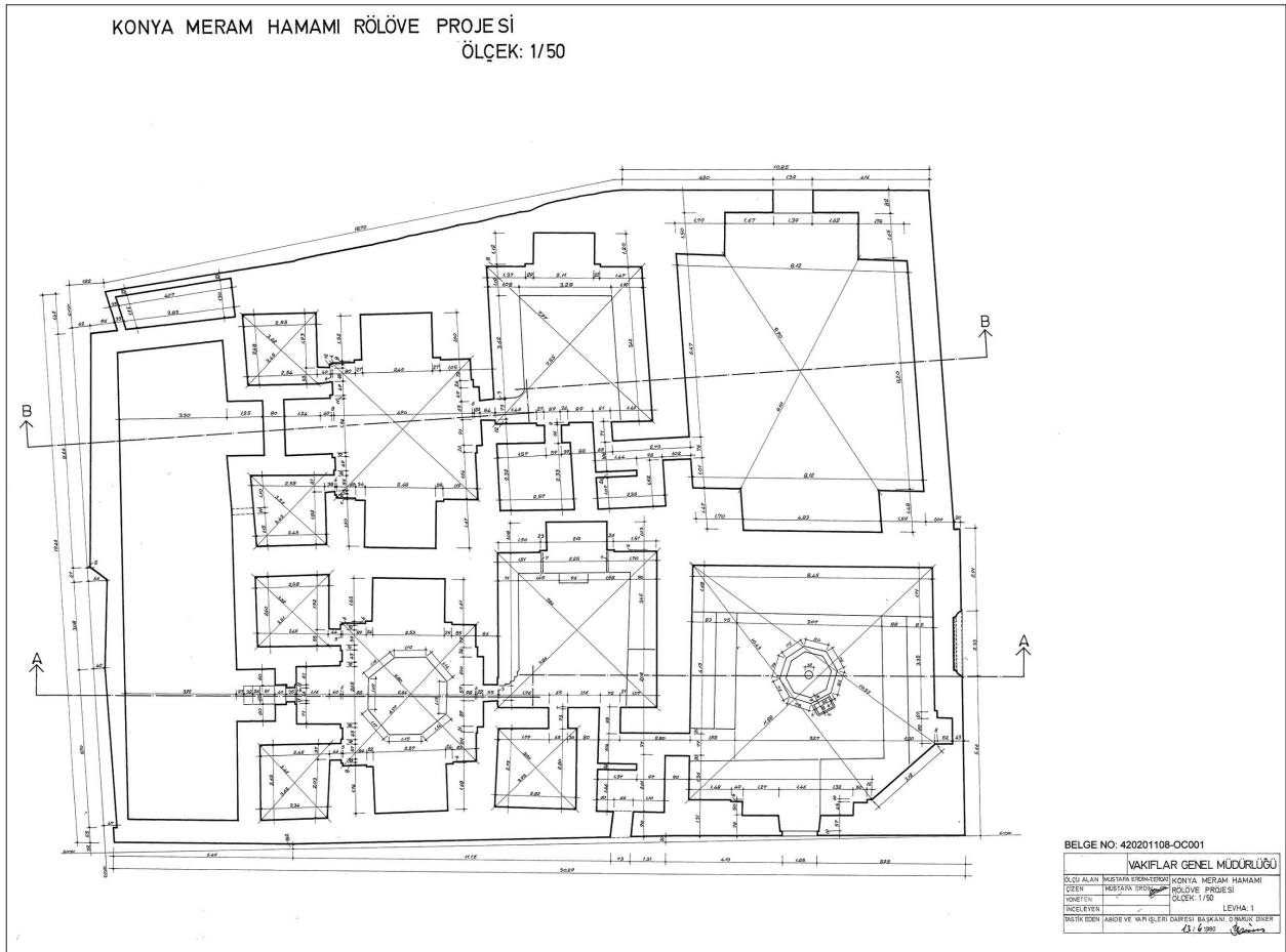
Şekil 8. Konya, Meram, Hatipoğlu/Hasbeyoğlu Hamamı (Proje Yöneticisi: Orhan Cezmi Tuncer Kaynak: Vakıflar Genel Müdürlüğü Arşivi, Meridien Envanter Programı, Konya, Meram, Hatipoğlu/Hasbeyoğlu Hamamı Dosyası)
