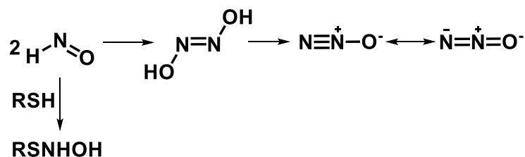
Schéme 19. Réactions de HNO en milieu aqueux ou biologique.
