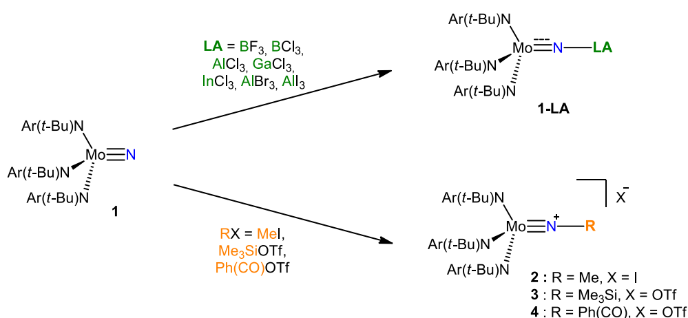
Schéma 1. Synthèse des adduits 1-LA et des complexes imido cationiques 2-4 .
