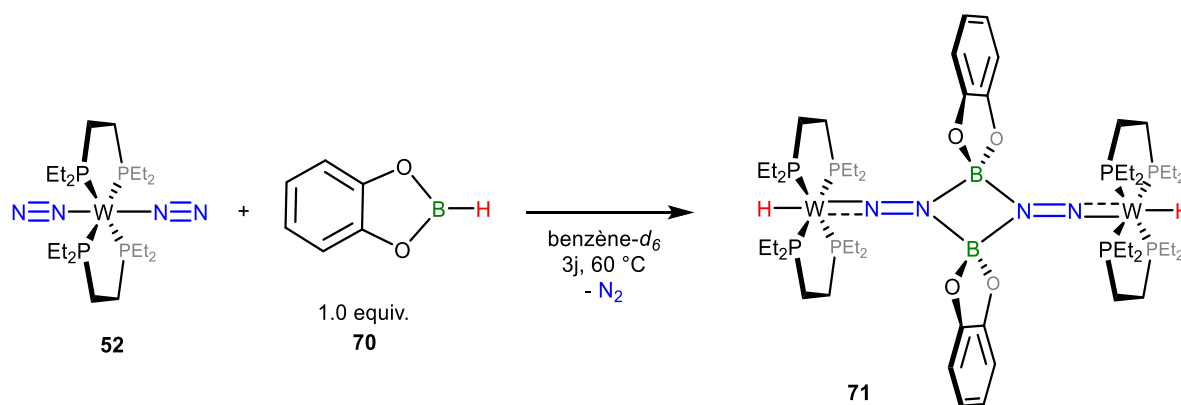
Schéma 27. Réaction entre le complexe trans -[W(N 2 ) 2 (depe) 2 ] ( 52 ) et le HBcat 70 .
