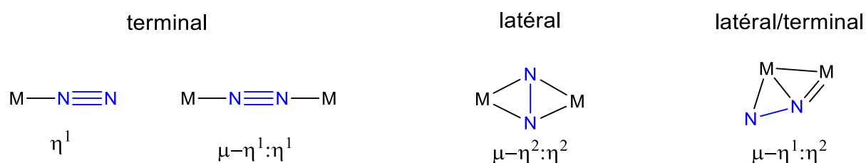
Figure 8. Modes de coordination du diazote à un métal.
