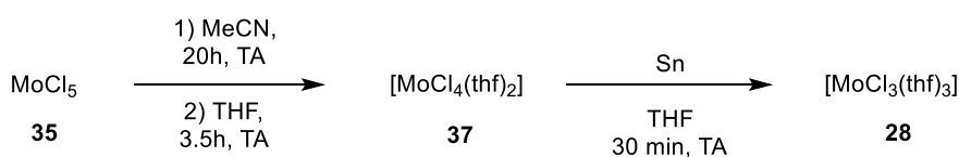
Schéma 8. Synthèse du complexe [\text{MoCl}_3(\text{THF})_3] ( 28 ).
