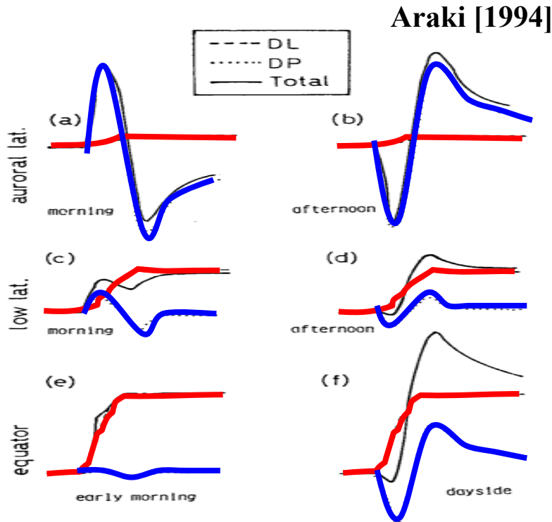
SC時に現れる磁場波形
