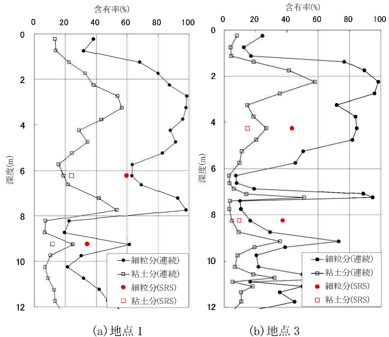
図-3 物理試験結果の深度分布(粒度)
