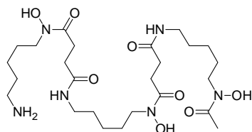
Desferrioxamine B (4)
