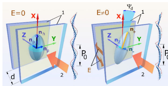
Рис. 2. Геометрия планарно-ориентированной ячейки DHFLC с равномерно закрученной спиралью: цифрой 1 обозначены стеклянные пластины, покрытые слоем оксида индия-олова (ИТО), поверх которых нанесены ориентирующие слои; стрелка 2 указывает направление распространения падающего линейно поляризованного света; d – толщина слоя DHFLC; P_0 – шаг спирали; n_p, n_h – показатели преломления спиральной структуры DHFLC при E = 0 [10]; \Psi_d(E) \sim E – отклонение главной оптической оси в электрическом поле
