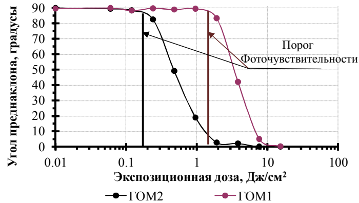
Рис. 2. Зависимость угла преднаклона от экспозиционной дозы для GOM1 и GOM2
