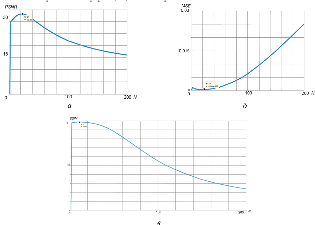
Рис. 2. Зависимость критериев оценки от количества итераций восстановлений: а – PSNR, б – MSE, в – SSIM
