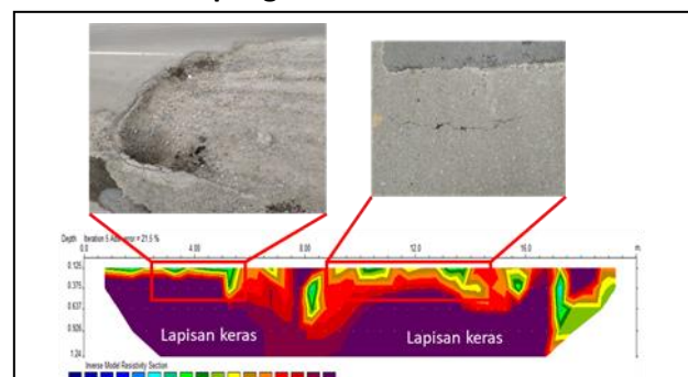
Gambar 7 Penampang resistivitas 2D Lintasan 1 (Bawah). Terlihat gambar kerusakan jalan (Atas)
