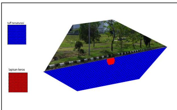
Gambar 1 Litologi Lintasan 3
