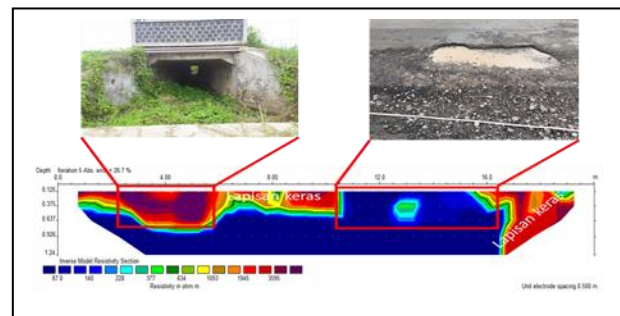
Gambar 9 Penampang resistivitas 2D Lintasan 2 (Bawah). Terlihat gambar kerusakan jalan dan keberadaan Tunnel air (Atas)
