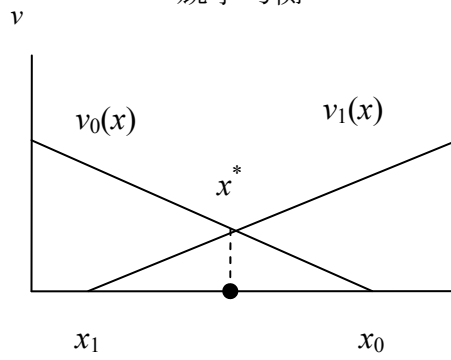
競争均衡
