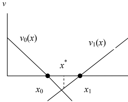
分離均衡
