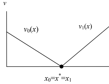
キンク均衡
