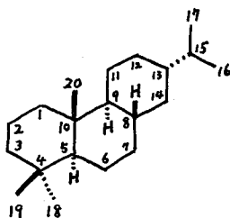
Abietane
