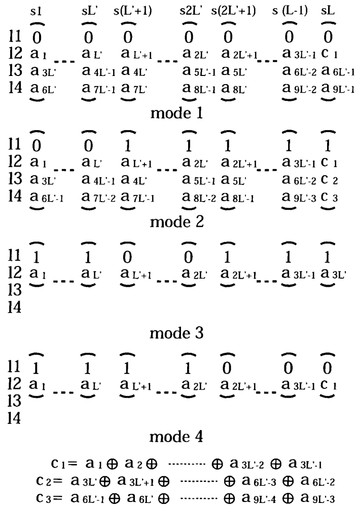
図 5.19: 4 モードの異なる伝送環境に対応したハイブリッド符号 (符号 5.3)
