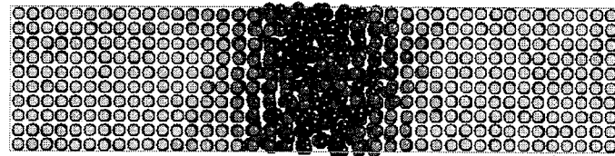
(b) 13000 step
