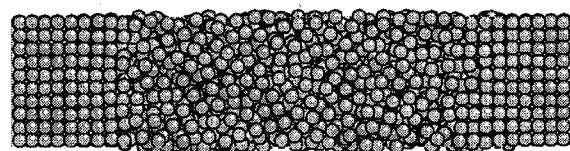
(b) 30000 step
