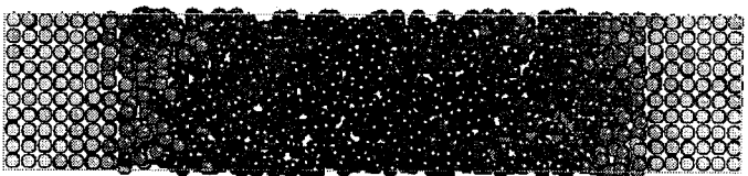
(e) 23000 step
