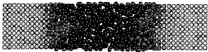
(d) 18000 step
