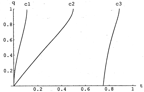
図 4.1 c_1, c_2, c_3 の解のグラフ
