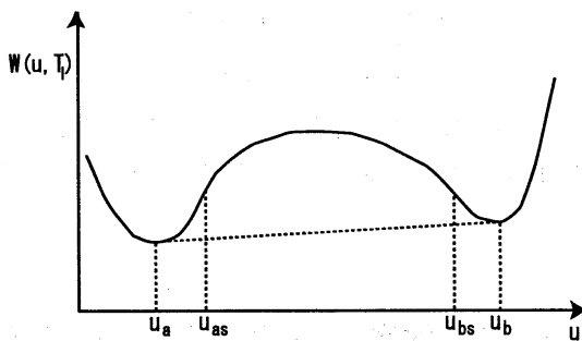
図 4: 自由エネルギー ( T < T_c )
