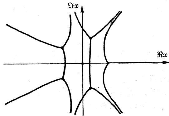
図 1-2. Q(x) = 1 - x^5
