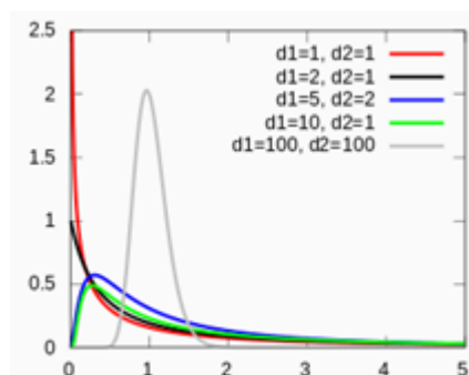
Figura 5. Funció de densitat de probabilitats de la distribució F. L'eix de les abscisses representa els valors possibles d'F i el de les ordenades la freqüència de cada valor. Els símbols d_1 i d_2 corresponen als dos graus de llibertat \nu_1 i \nu_2 . S'observa que al augmentar els graus de llibertat la distribució és més propera a la distribució de Laplace-Gauss.
