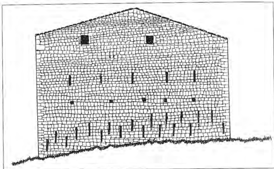
Casa del Port de Sant Isclé de Colltort. Façana (B).
