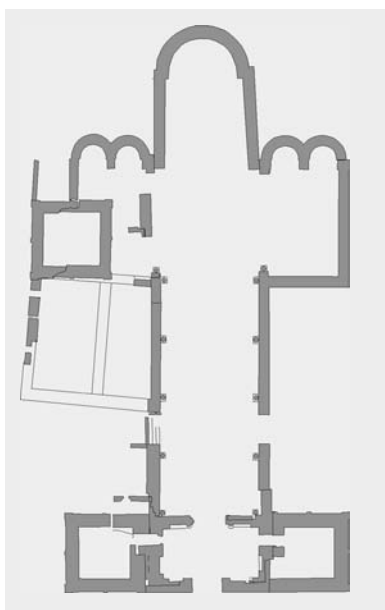
Planta de la catedral romànica de Girona.
