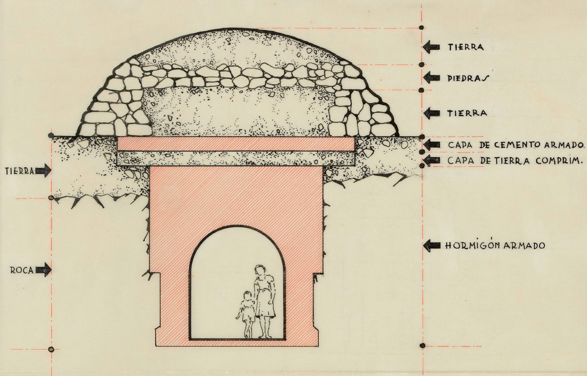
SECCIÓN del REFUGIO ESCALA 1:50
