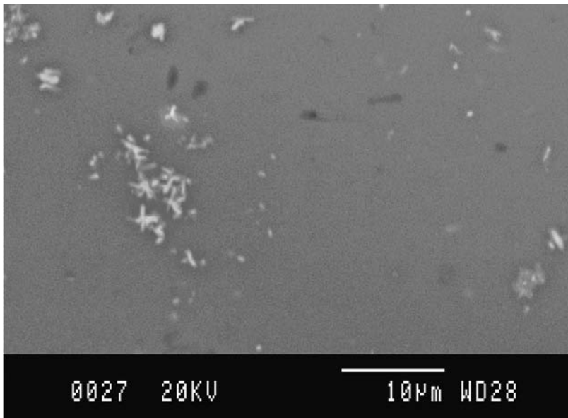
Figura 5.1 Microfotografia realitzada per MER-ES del Ic DIA643, en la que es poden apreciar en gris clar els cristalls d'òxid d'estany (SnO2) dispersos en el vidrat.
