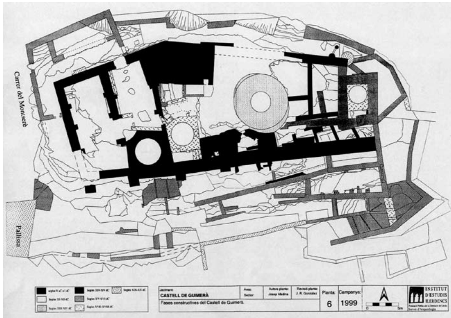
Fig. 1. Plànol de la planta del castell de Guimerà després de les excavacions, amb tota la planimetria i els detalls de les fases de la seva construcció, la base de la torre i els tres cups de vi. J.F. Medina Morales, Serveis d'Aqueologia, IEI, Lleida, 1999.
