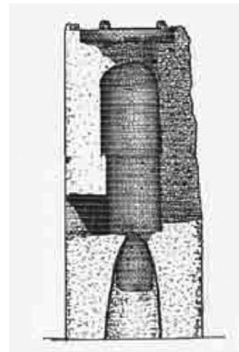
Fig. 9. Tall de la torre de guaita on s'observen les parts de l'edifici així com l'espai de la zona que feia de magatzem i també de possible presó, a la base de la qual es localitzaren un grafit ibèric. Dibuix M.A. Corbella.
