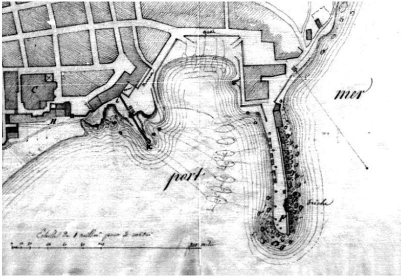
El moll vell de Palamós construït pel duc de Sessa a principis del segle XVIII en un plànol francès de 1823.
