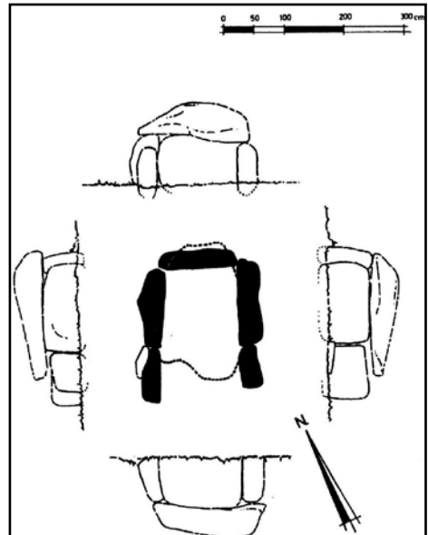
Planta i seccions del sepulcre (Roca et al. , 1980: 26, Fig.1).
